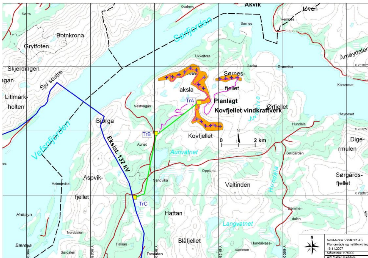
Figur 7: Kovfjellet vindkraftverk med nettilknytning
