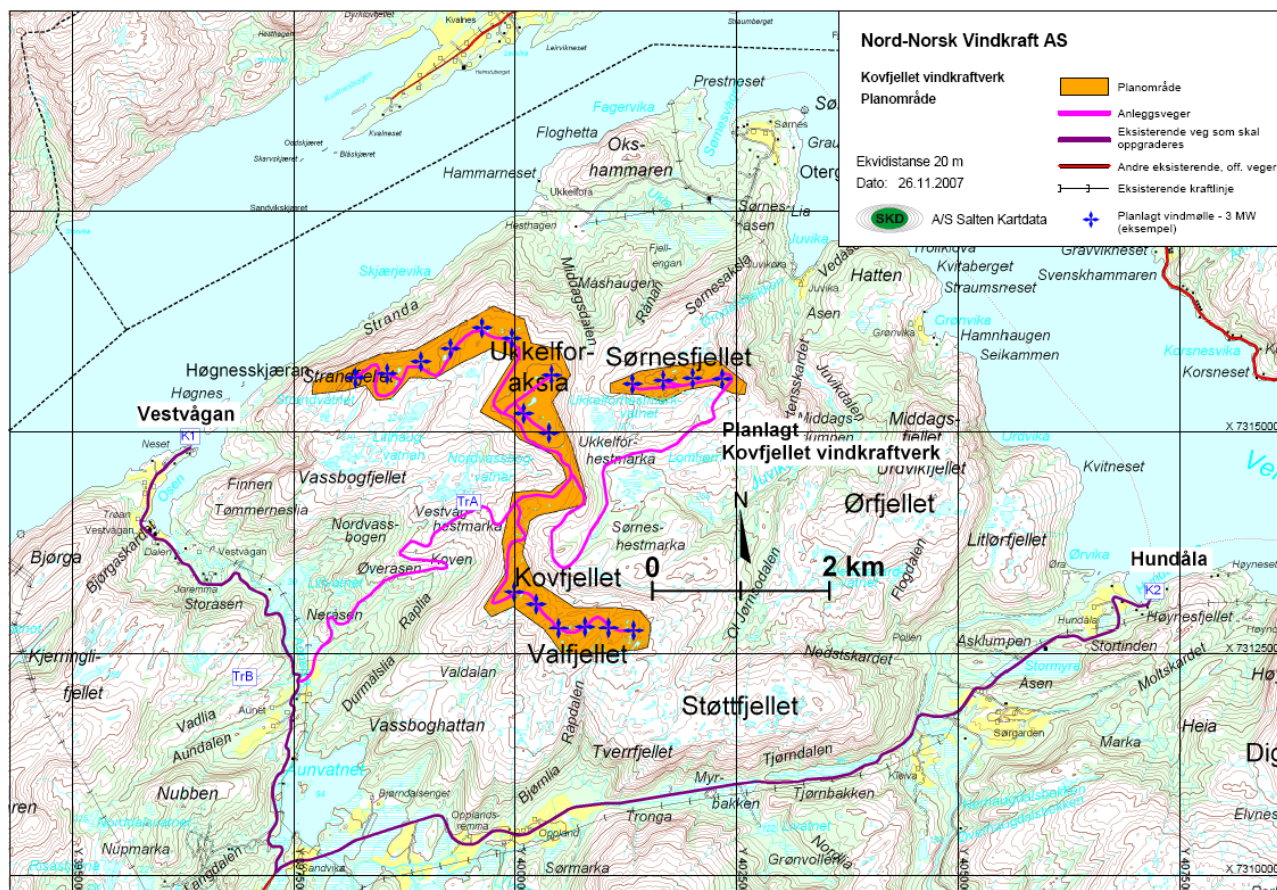
Figur 5: Planområde Kovfjellet vindkraftverk med inntegnet eksempel for 3 MW vindmøller
