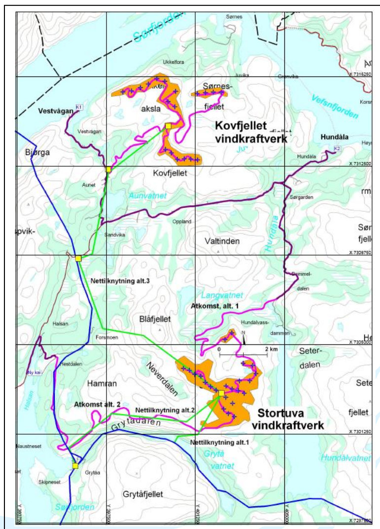
Figur 6: Innbyrdes plassering av Stortuva vindkraftverk og Kovfjellet vindkraftverk
