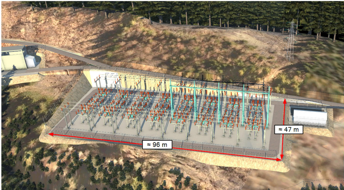
Figur 3 Omsøkt 132 kV koblingsanlegg.
