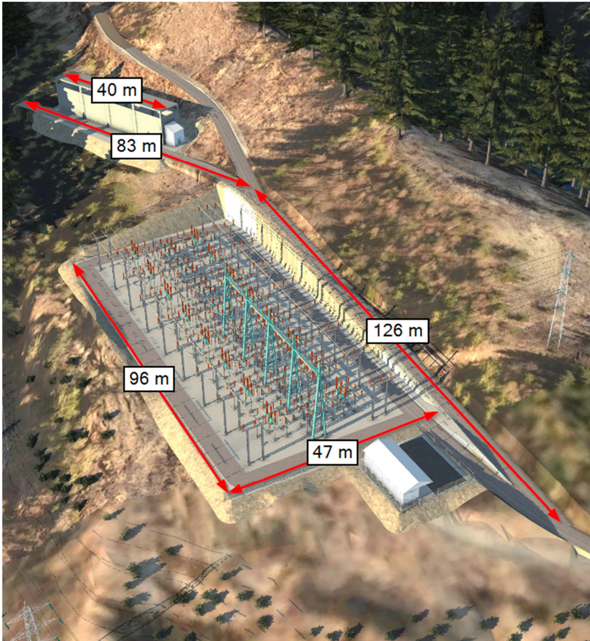
Figur 2 Nærbilde av omsøkt anlegg. 132 kV koblingsanlegg i front, nye transformatorer i bakkant.
