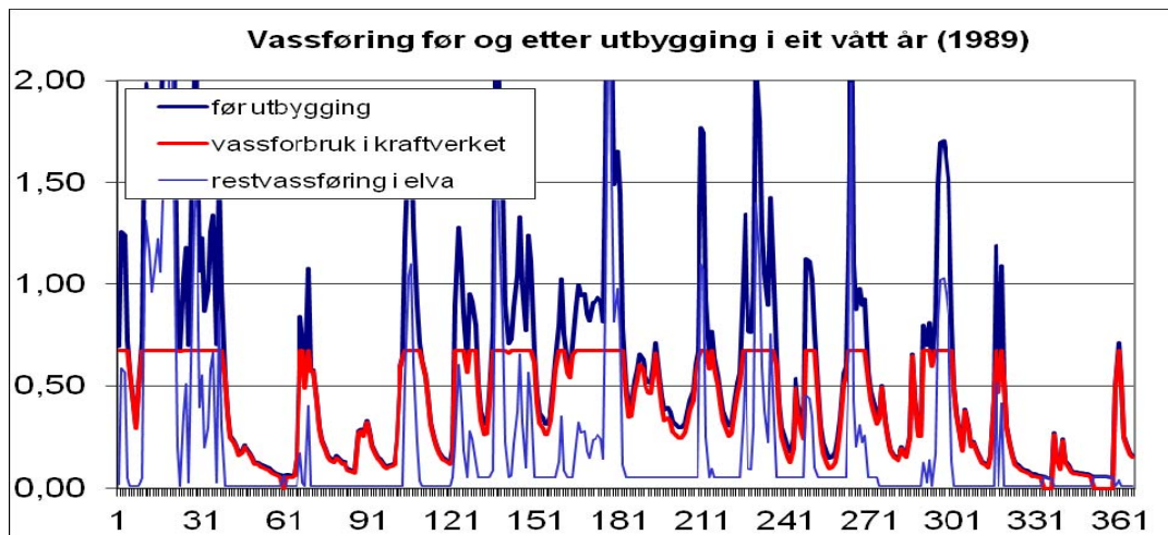
Figur 8. Plott som viser vannføringsvariasjoner i et vått (1989) år (før og etter utbygging). 18
