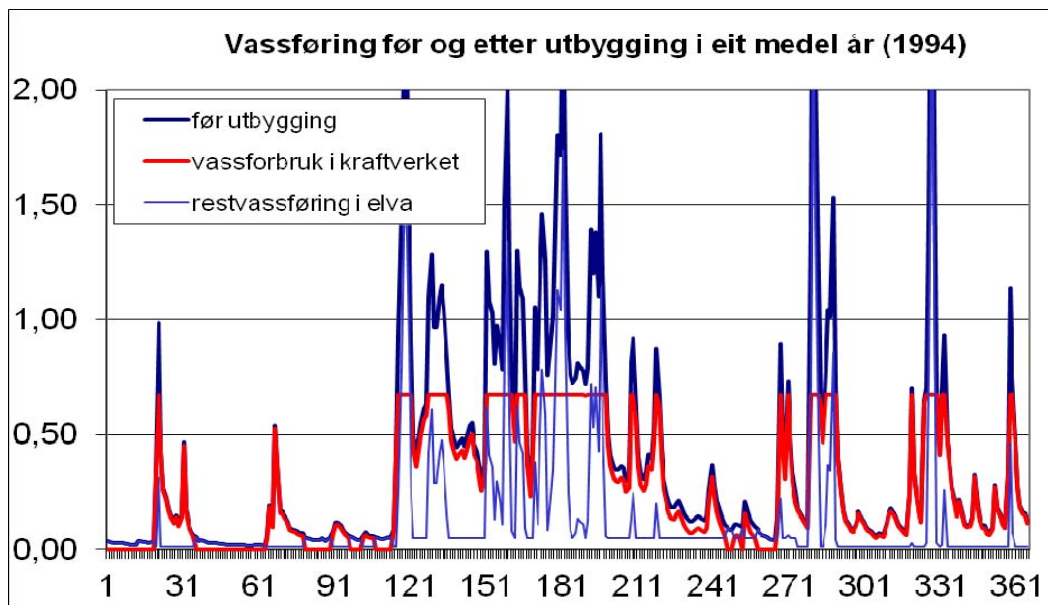
Figur 7. Plott som viser vannføringsvariasjoner i et middels (1994) år (før og etter utbygging). 17
