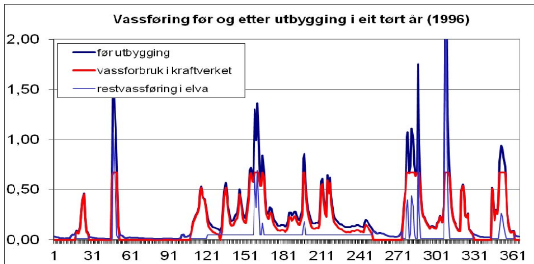
Figur 6. Plott som viser vannføringsvariasjoner i et tørt (1996) år (før og etter utbygging). 16
