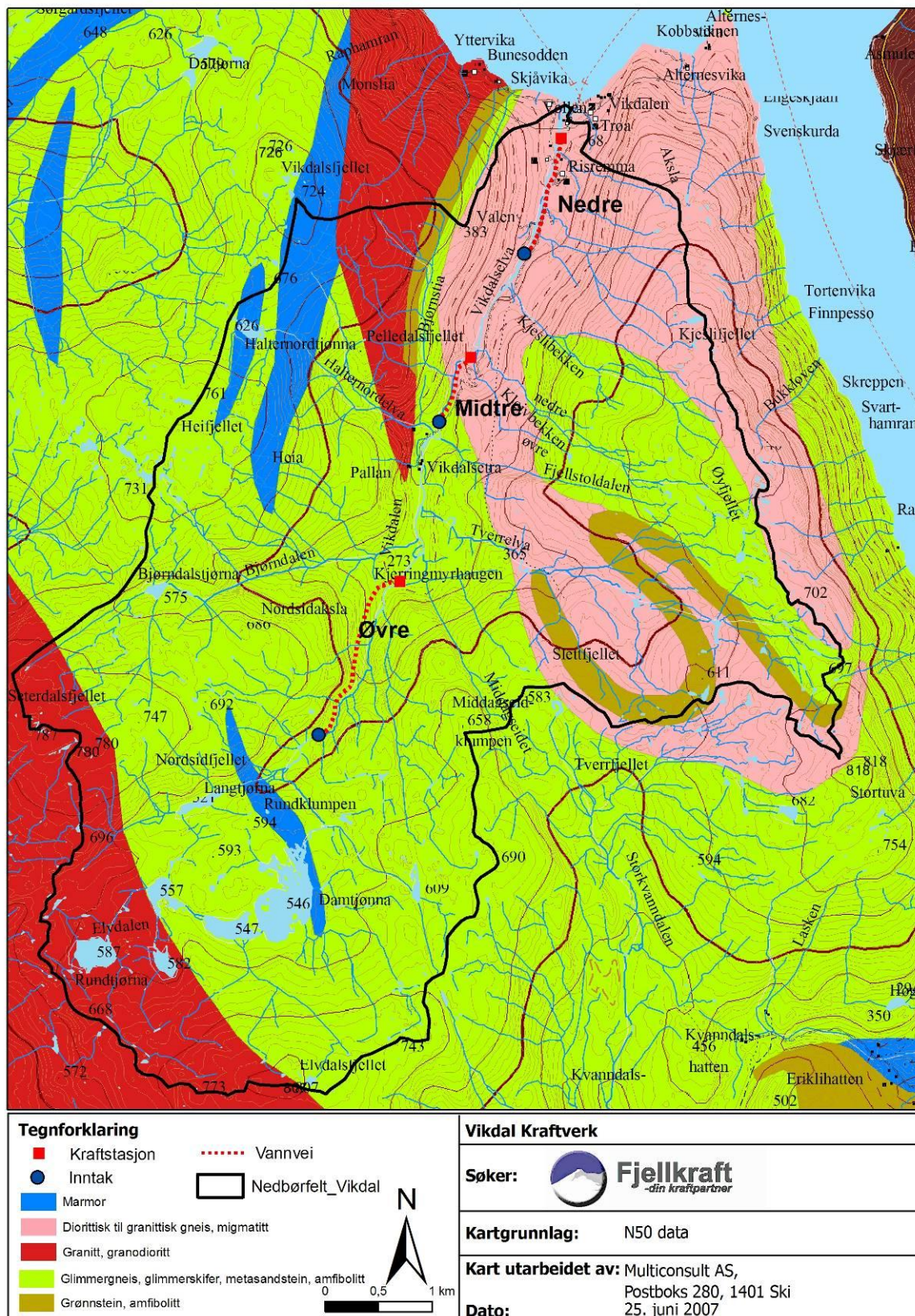
Figur 1. Berggrunnsgeologien i Vikdalen og omkringliggende områder. Midtre Vikdal kraftverk samt to kraftverk planlagt oppstrøms og nedstrøms (ikke utredet her) er inntegnet.
