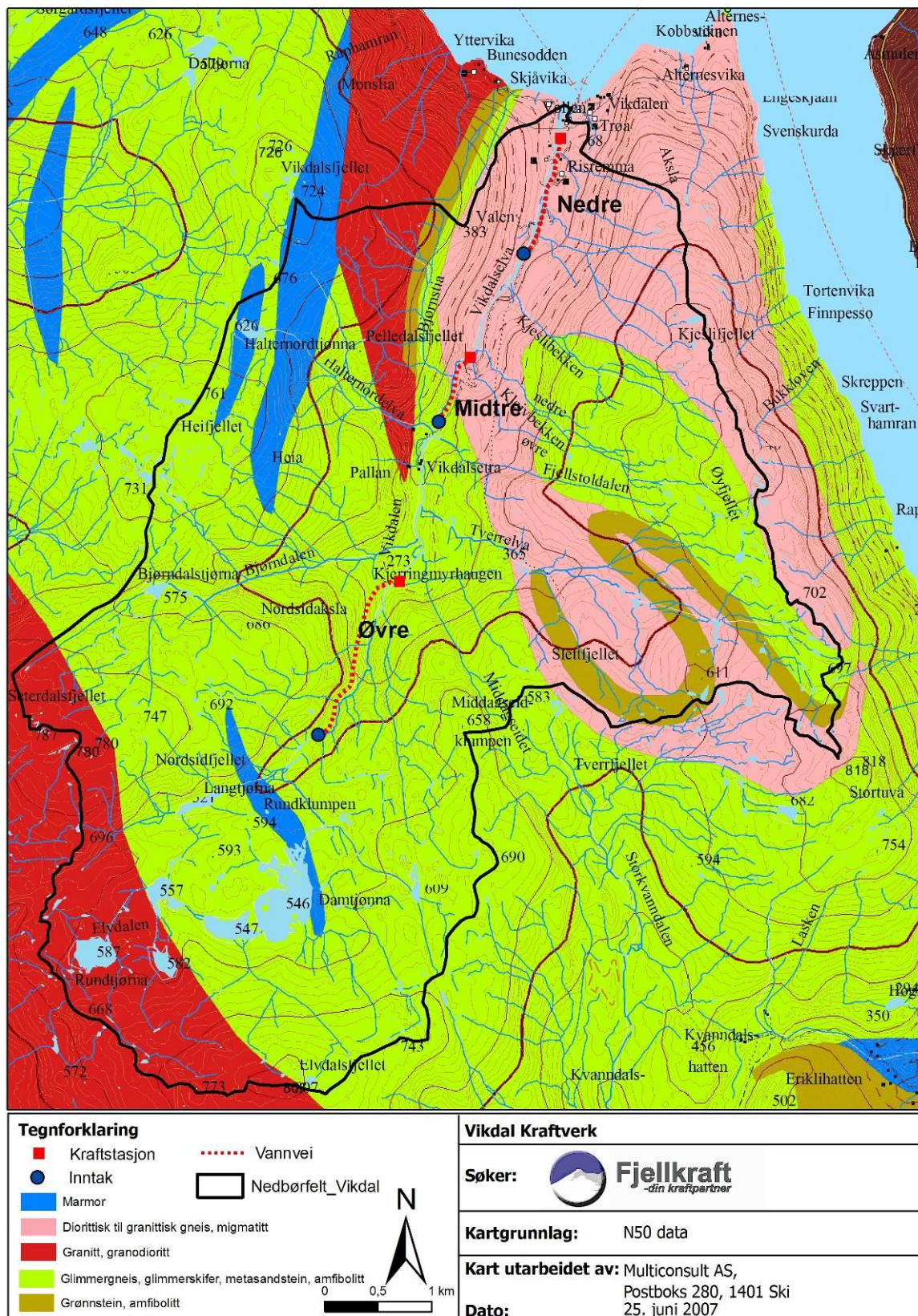
Figur 2. Berggrunnsgeologien i Vikdalen og omkringliggende områder. Nedre Vikdal kraftverk samt to kraftverk planlagt oppstrøms (ikke utredet her) er inntegnet.
