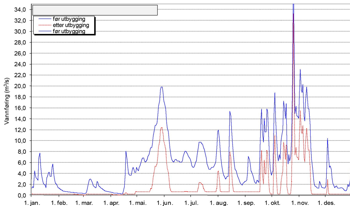
Sæverhagen kraftverk. Vannføring nedenfor inntaket - vått år - 1983
