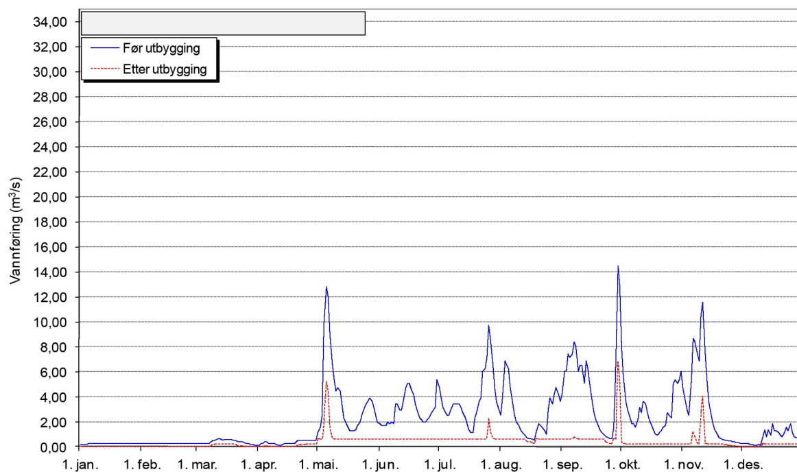
Sæverhagen kraftverk. Vannføring nedenfor inntaket - tørt år - 1977
