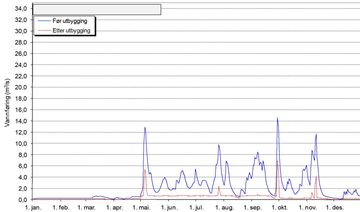
Sæverhagen kraftverk. Vannføring ovenfor utløpet - tørt år - 1977
