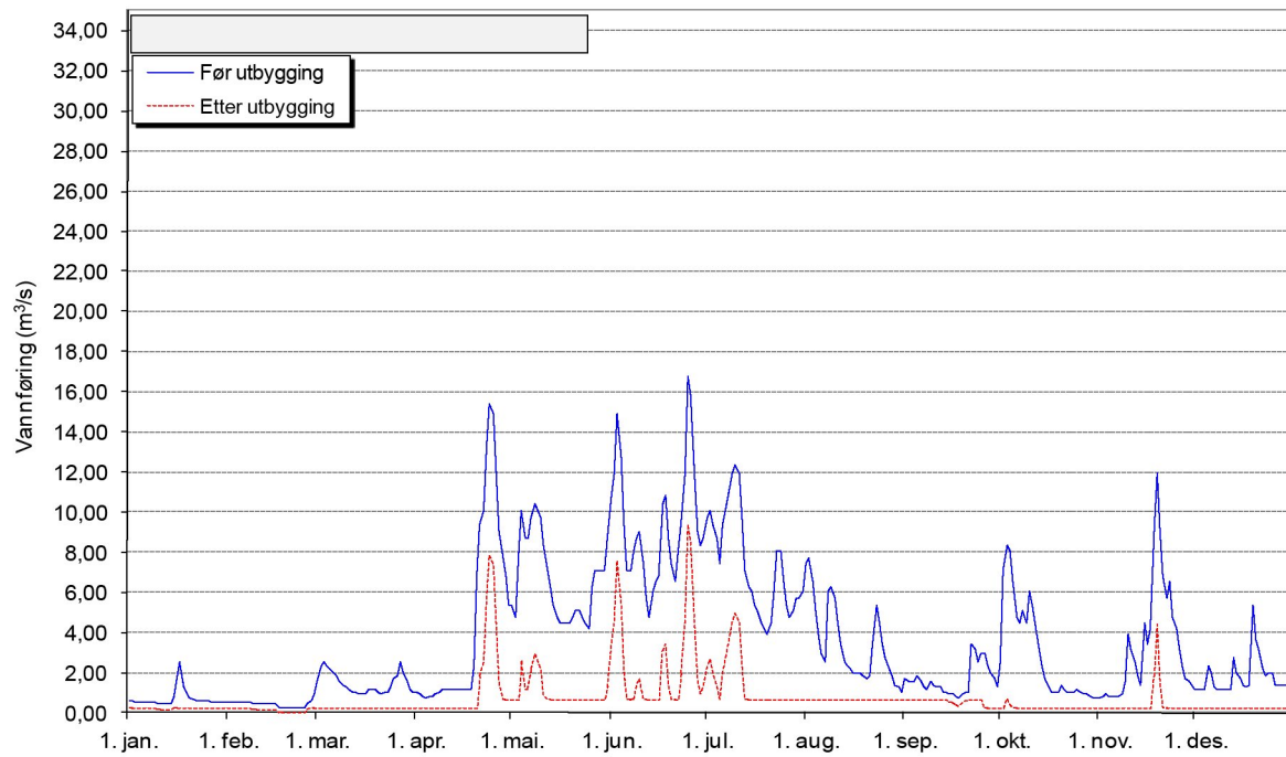
Sæverhagen kraftverk. Vannføring nedenfor inntaket - middels år - 1994
