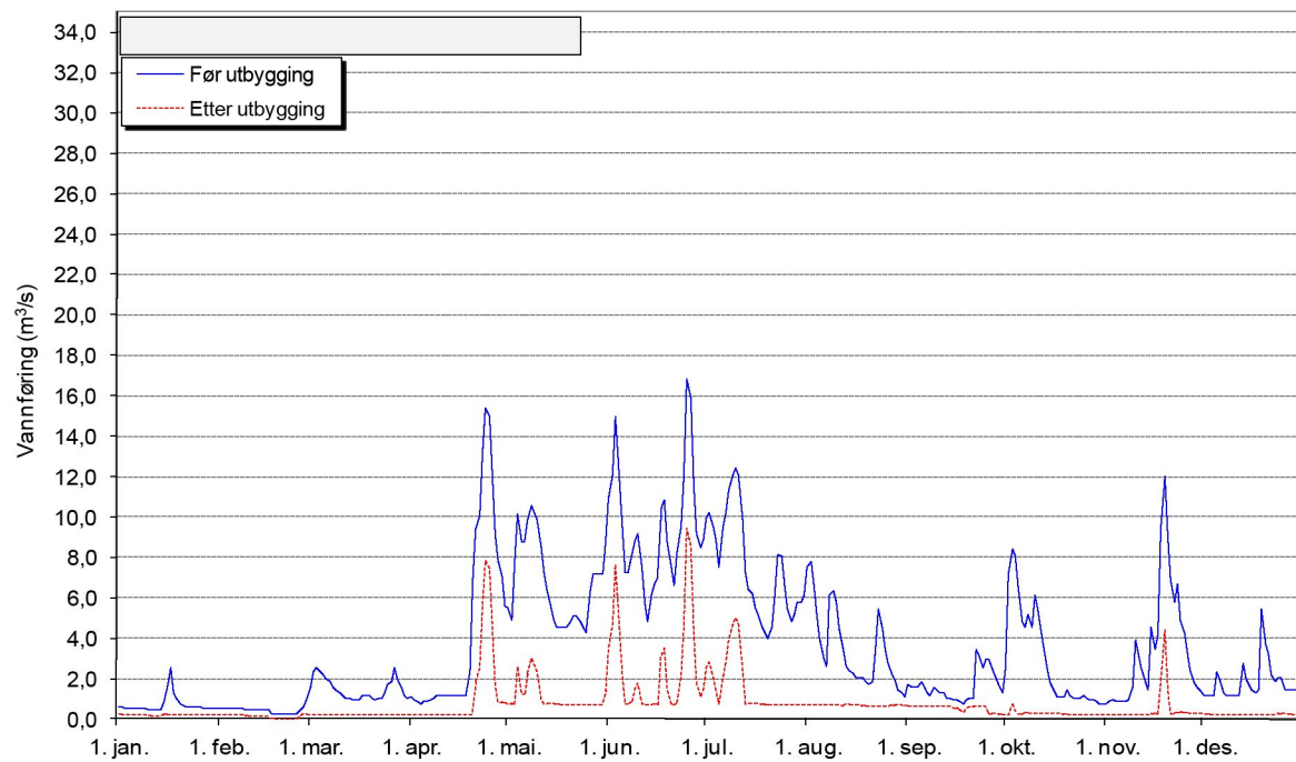
Sæverhagen kraftverk. Vannføring ovenfor utløpet - middels år - 1994
