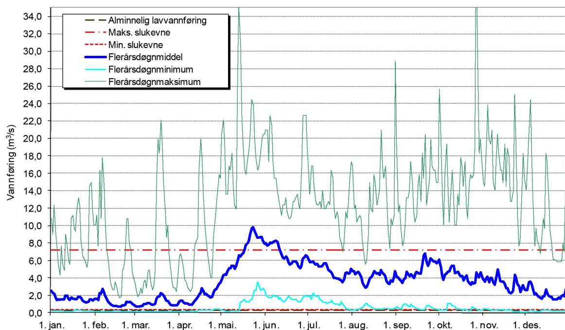
Sæverhagen kraftverk. Vannføring nedenfor inntak, flerårsstatistikk før utbygging, 1976 - 1994
