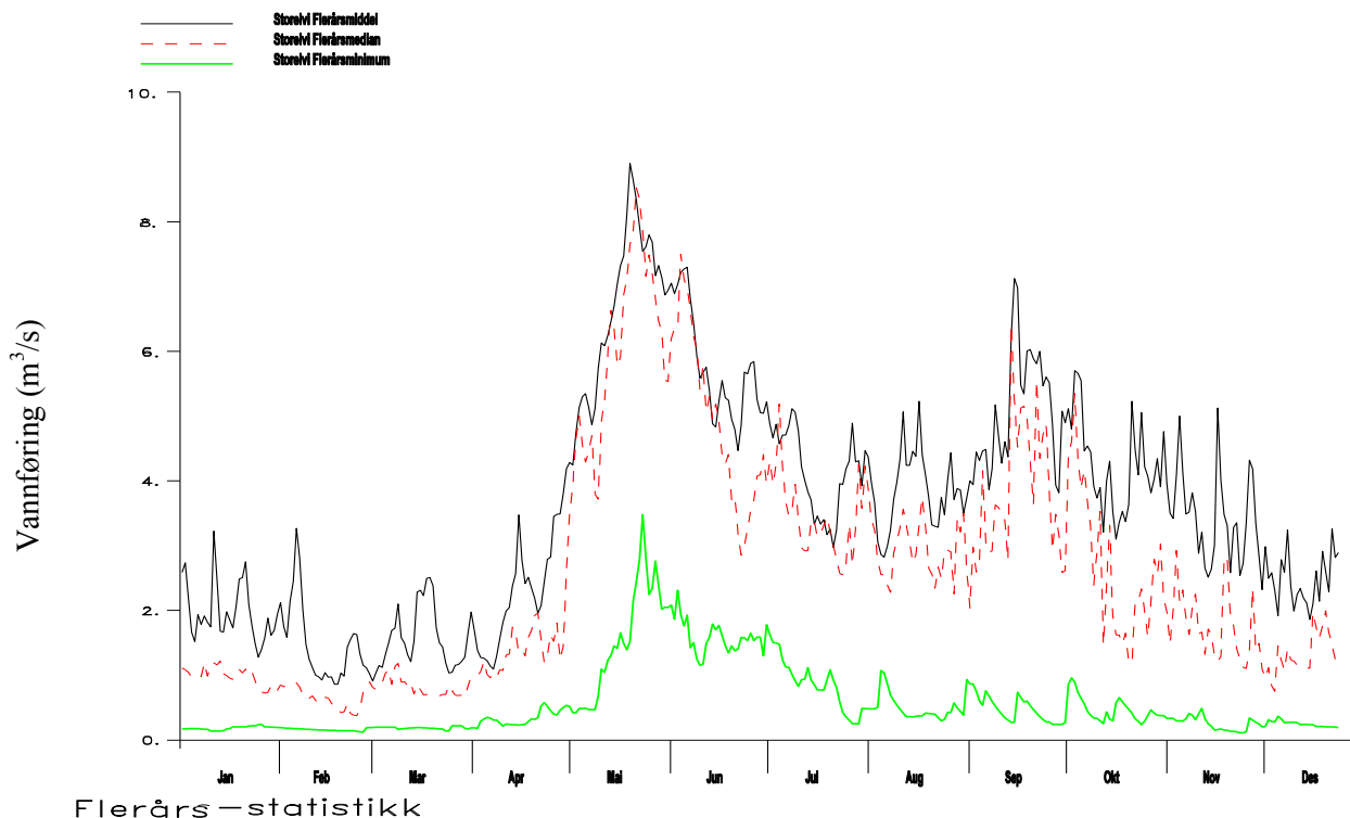
Figur 4. Kurven viser sesongvariasjonen i vannføringen i \text{m}^3/\text{s} i Storelvi basert på flerårs døgnverdier. Flerårsmiddel, flerårsmedian og flerårsminimum er presentert. Sesongvariasjonene er antatt å samsvare noenlunde med kombinasjon av nedbørfeltene til målestasjonene 47.7 Fodnastøl og 42.2 Djupevad.
