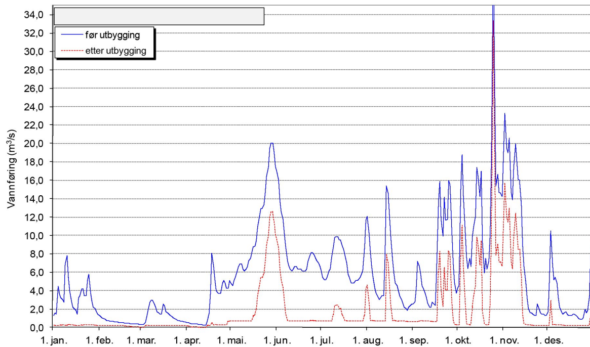
Sæverhagen kraftverk. Vannføring ovenfor utløpet - vått år - 1983
