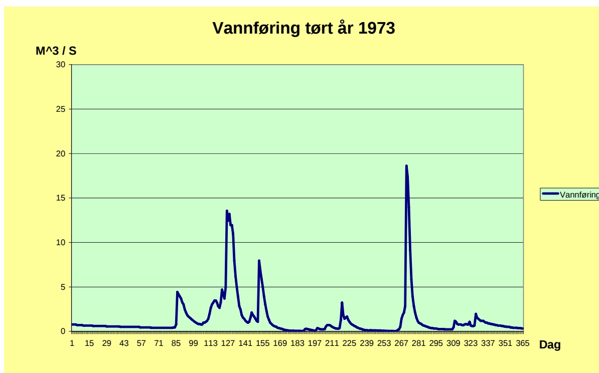
Figur 6. Plott som viser vannføringsvariasjoner i et tørt år (1973). 16
