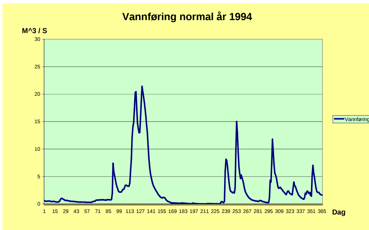
Figur 7. Plott som viser vannføringsvariasjoner i et middels år (1994). 17
