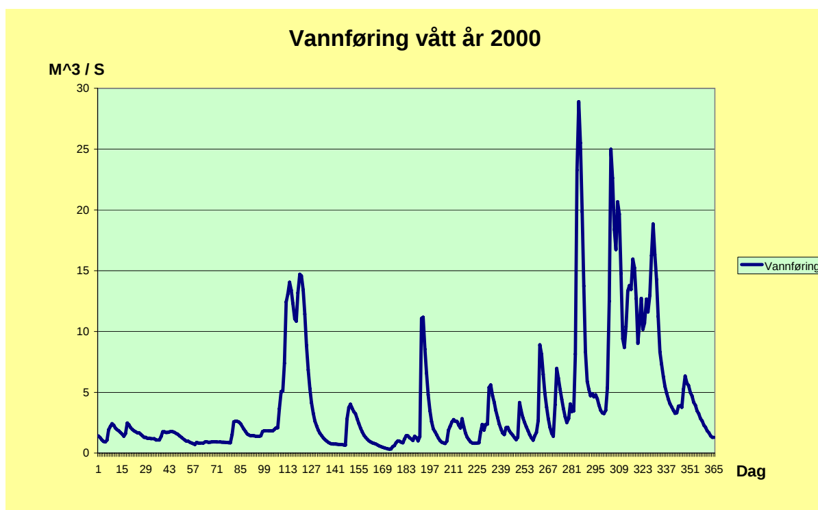
Figur 8. Plott som viser vannføringsvariasjoner i et vått år (2000). 18
