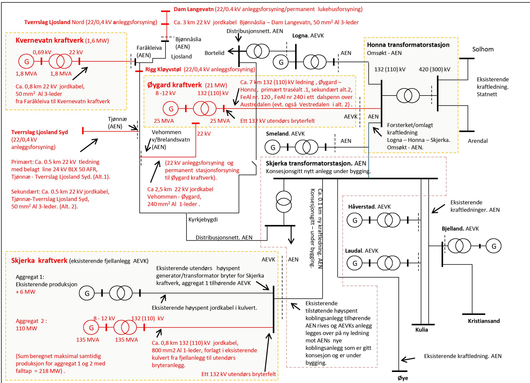
Vedlegg 16. Oversikt konsesjonssøkt nettløsning - Åseral prosjektene - AEVK. Rød = konsesjonssøkt - AEVK. Tegning AEVK.
