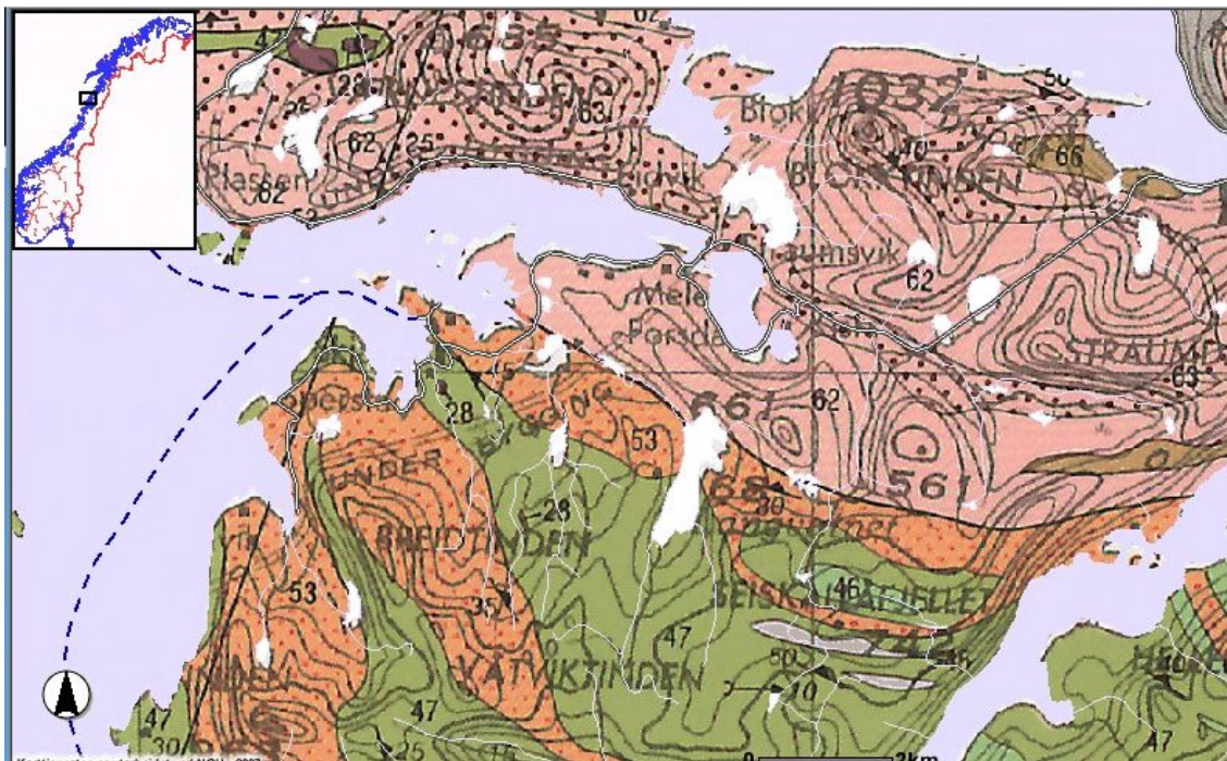
Figur 6. I utbyggingsområdet finner en nesten bare harde og sure bergarter som ymse gneisarter, slik som det rosafargede området i nordenden av kartutsnittet (62). Den grønne fargen (47) som dominerer i den sørlige delen består i hovedsak av glimmergneis og glimmerskifer, bergarter som regnes som litt mindre fattig enn ren gneis, mens en i det midterste partiet (den oransjefargede fargen 53) der de fleste inngrepene eventuelt vil bli foretatt, også finner gneiser, her med granittisk til tonalittisk sammensetning. (Gustavson & Gjelle 1991. NGU 2007).
