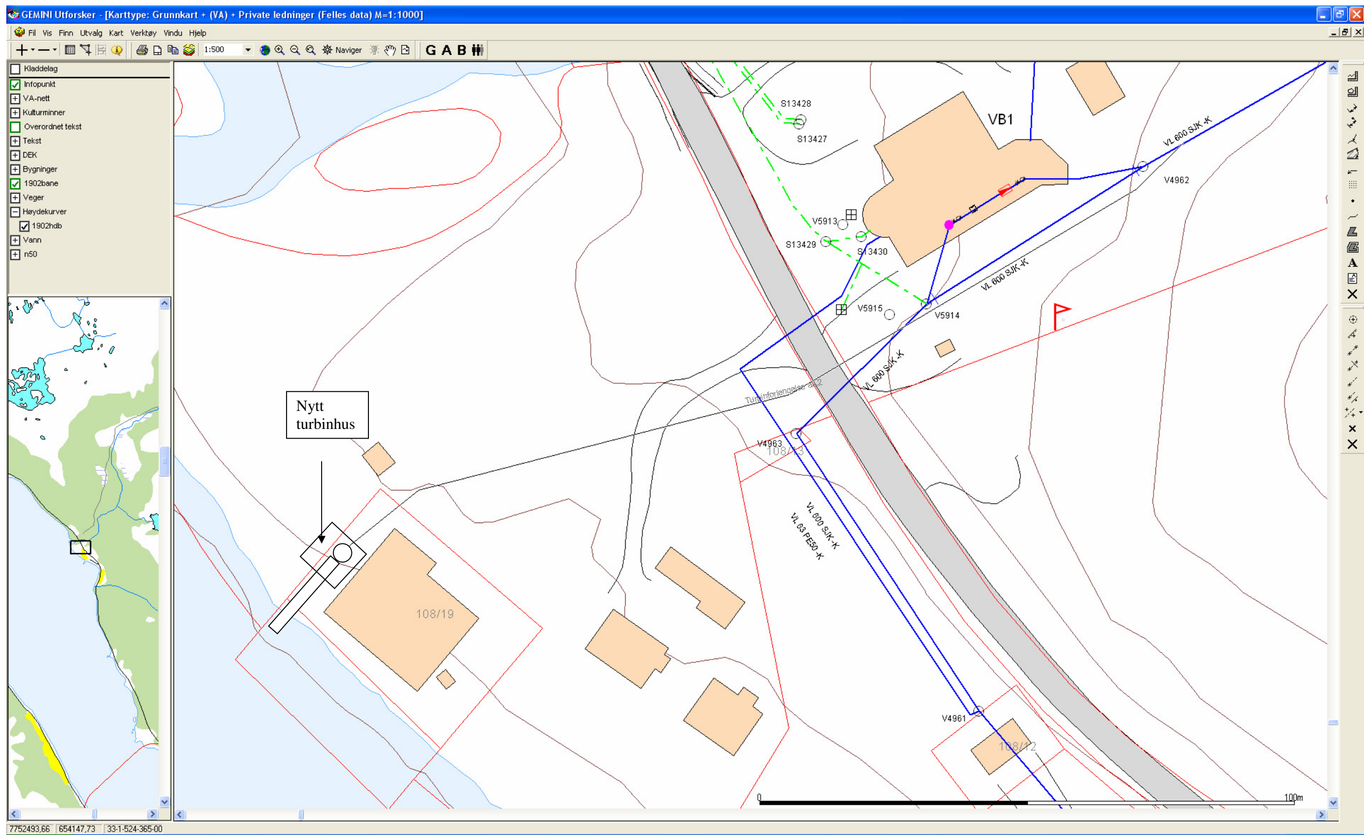
Figur 11 (1:500 alt. 2 turbinrør forlengelse til nytt turbinhus)
