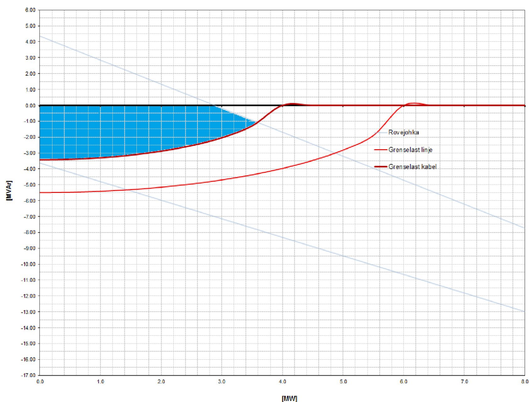
Figur 1 Krav til reguleringsområde som funksjon av aktiv produksjon ved Rovejohka i Storfford kommune
