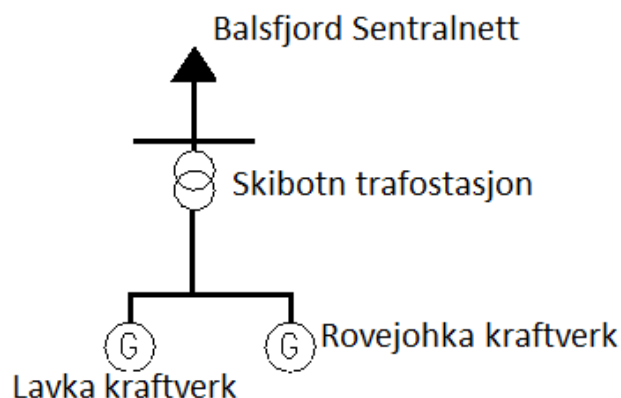
Figur 2 Enlinjeskjema for avgang fra Skibotn trafostasjon
