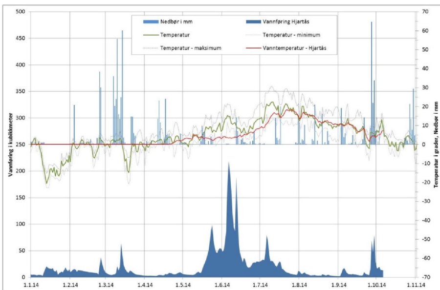
Figur 3.1. Nedbør i mm (lys blå), døgnmiddel lufttemperatur (grønn) med oppgitt maksimum og minimum (grå), og døgnmiddelvannføring (rød) og døgnmiddelvannføring i Ranelva målt ved terskelen oppstrøms Raufjellforsen i perioden 1.1.2014 til 06.10.2014.
