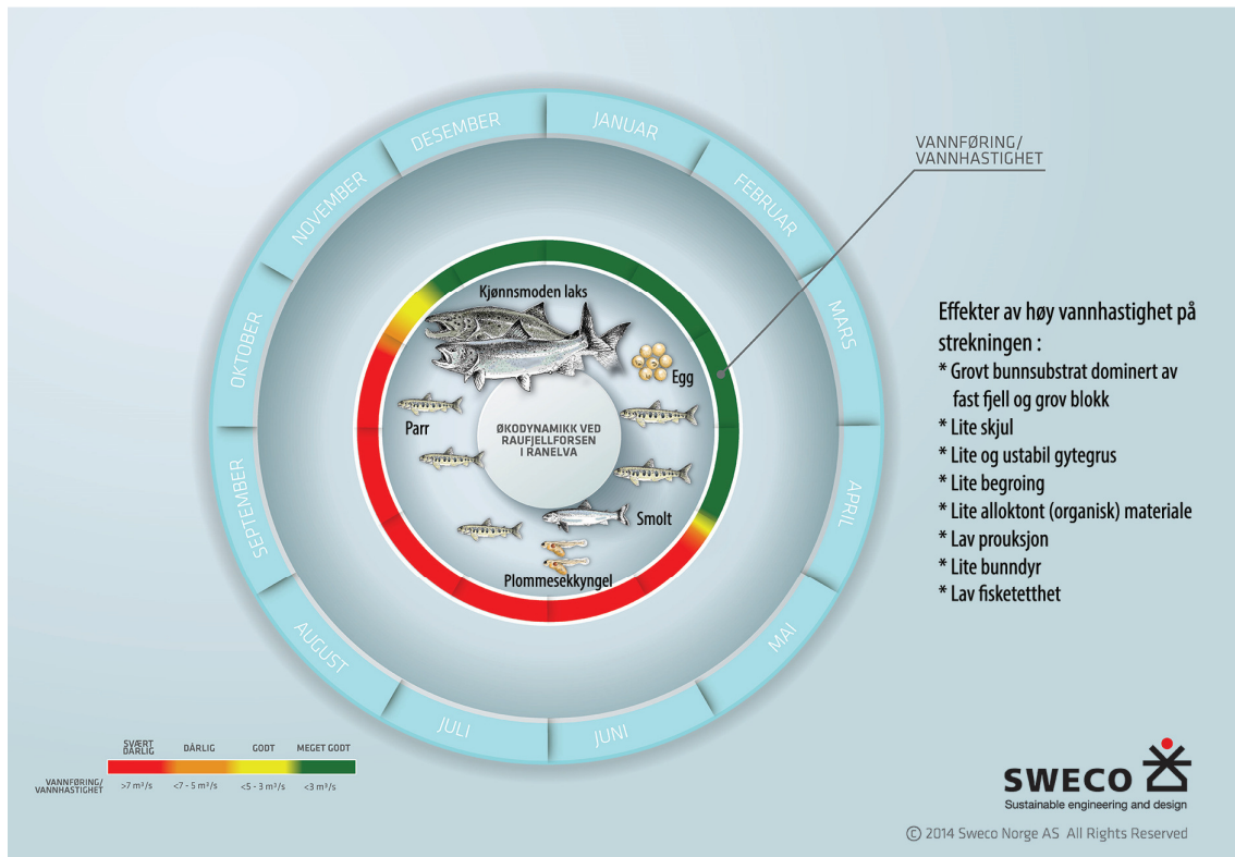
Figur 5.4. Årsvariasjonen i vannføring / vannhastighet for elvestrekningen i Ranelva i Raufjellfossen og ned til samløpet med Bjellåga, med inndeling i periodene svært dårlig (rød; vannføring > 7 m 3 /s), dårlig (oransje; vannføring <7 – 5 m 3 /s), god (gul; vannføring <5 – 3 m 3 /s) og svært god (grønn; vannføring < 3 m 3 /s). Tegningene av kjønnsmoden laks, egg, plommesekeyngel, parr og smolt viser en forenklet livssyklus i ferskvann og når på året de opptrer. Parren er i elva i flere år og er derfor tegnet inn flere steder i forhold til årshjulet. Tegninger av fisken: Finn R. Gravem.
