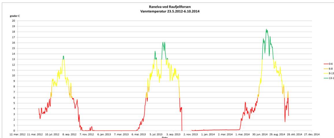
Figur 5.2. Vanntemperatur (døgnmiddel) målt ved terskelen der jernbanen krysser Ranelva oppstrøms Raufjellfossen i perioden fra 24.05.2012 til 6.10.2014. Rødt angir vanntemperaturen mellom 0 og 6 °C, oransje mellom > 6 og 8 °C, gult mellom > 8 og 13 °C og grønt > 13 °C. Inndelingen av temperaturkurven i ulike farger tilsvarer de intervallene som siden er benyttet til å vurdere de økodynamiske forholdene for den aktuelle elvestrekningen.
