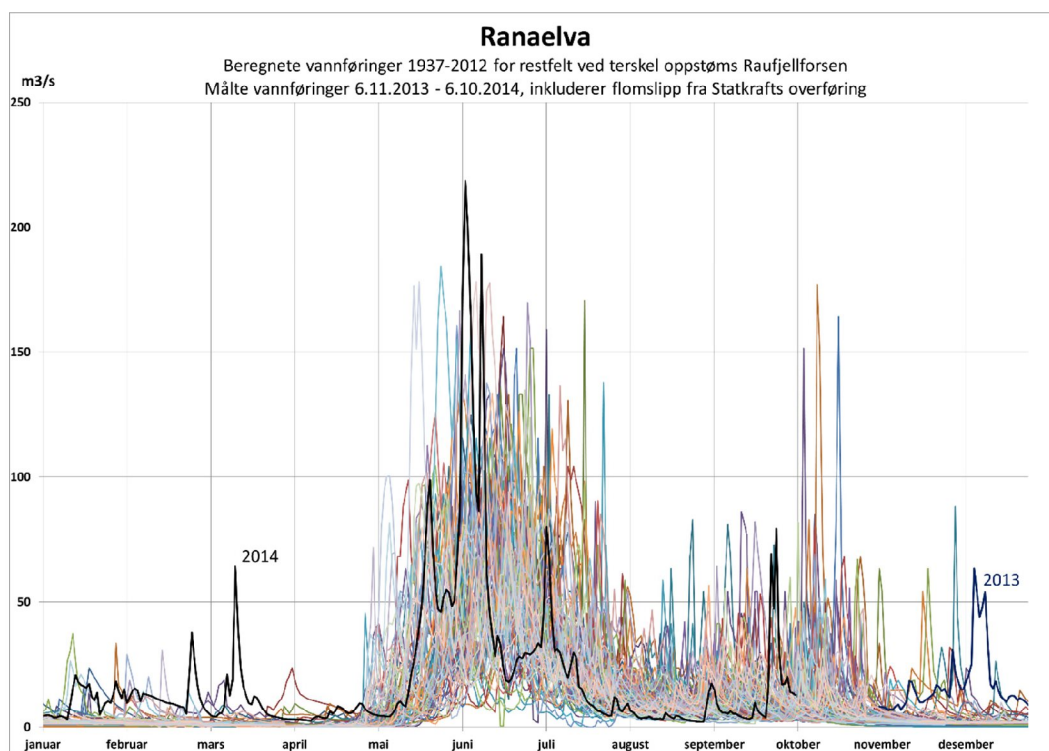
Figur 4.34. Beregnede vannføringer i Ranelva gjennom året oppstrøms terskelen (planlagt inntak for Hjørtås kraftverk) for perioden 1937 – 2012, og målte vannføringer for 2013 (rød kurve) og 2014 (sort kurve). Disse to årene har ikke fullstendige måleserier. De beregnede vannføringene tar ikke hensyn til flomoverløp fra Statkrafts overføringer, noe som er inkludert i vannføringskurvene fra 2013 og 2014. Hver enkelt kurve med sin farge representerer et år, og summen av alle kurvene gjenspeiler variasjonen som har funnet sted i vassdraget for angitte periode.
