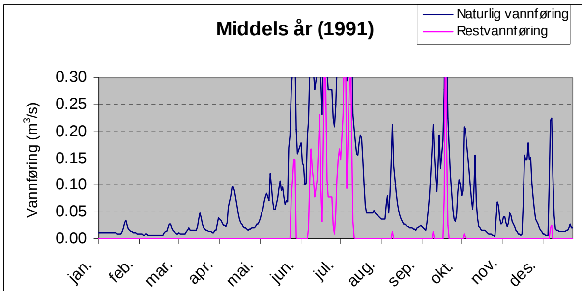
Figur 8.1 Plott som viser vassføringsvariasjonar Botnagrovi i eit middels (1991) år (før og etter utbygging). 17
