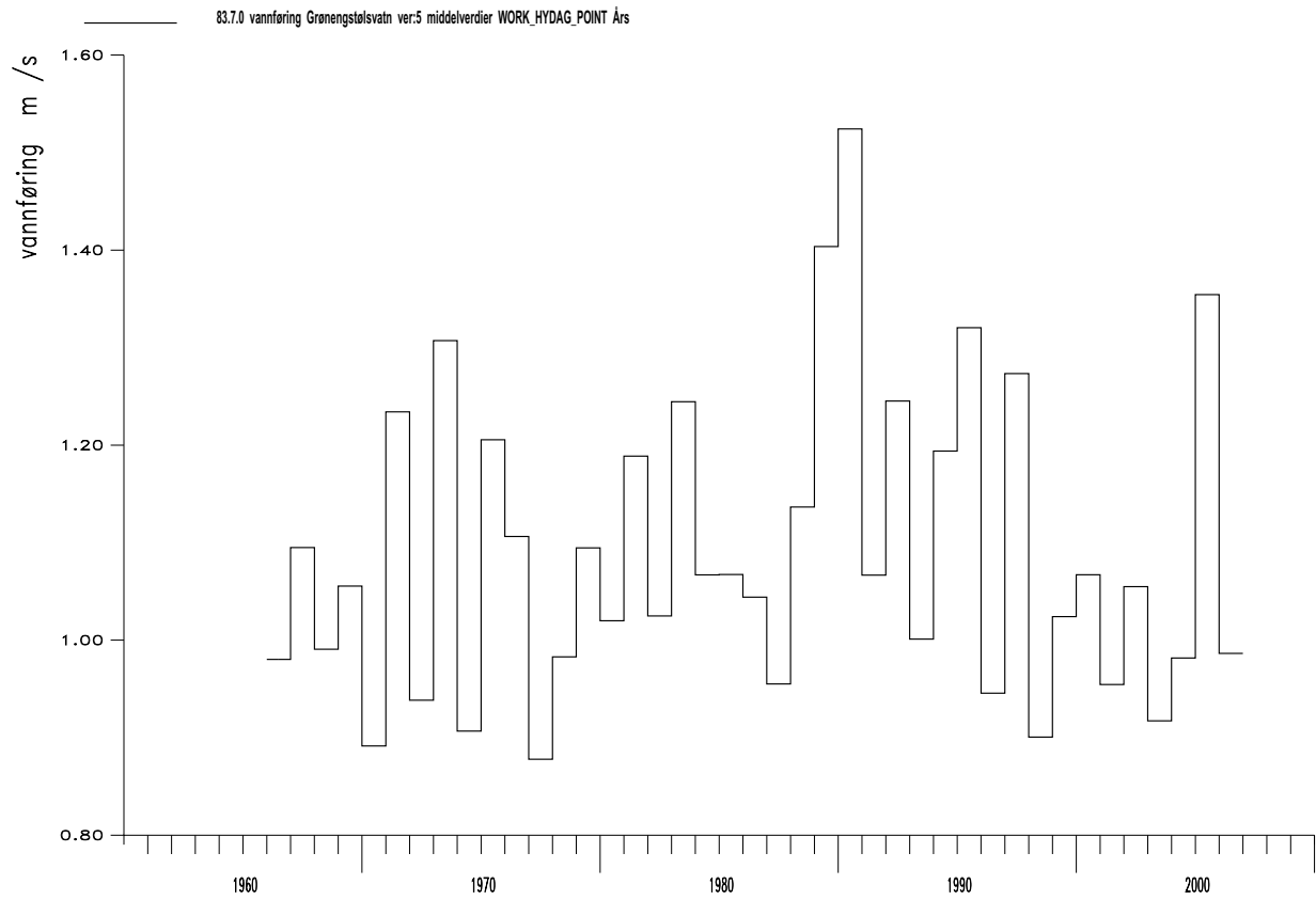
Figur 5. Plott som viser variasjoner i vannføring fra år til år. Vassføring i m 3 /s.
