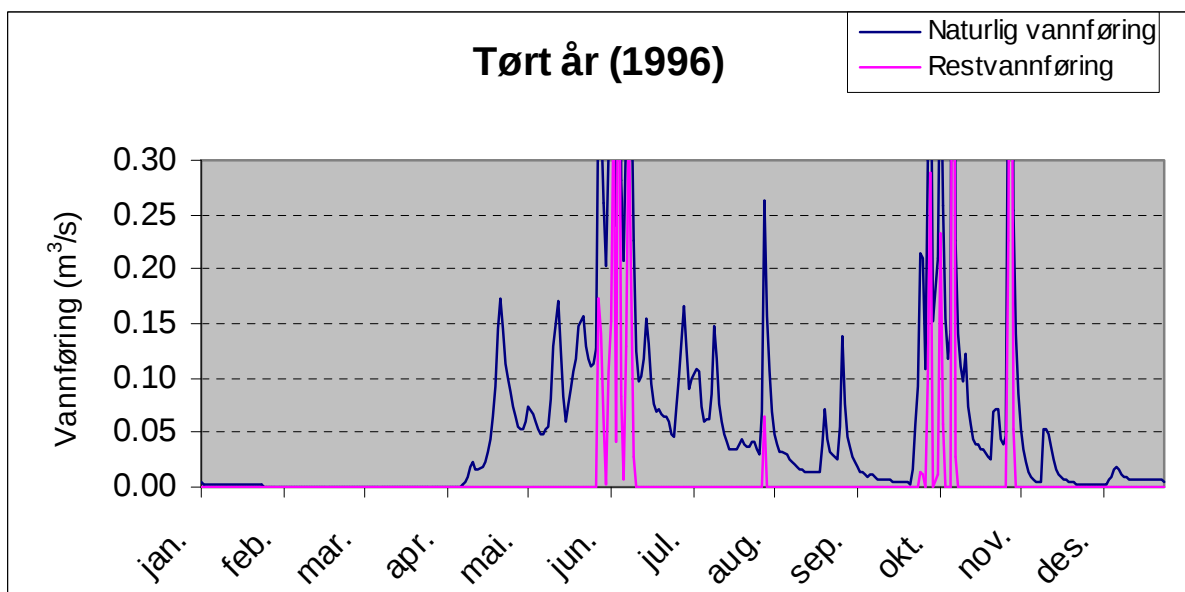
Figur 6.1 Plott som viser vassføringsvariasjonar i Botnagrovi i eit turt (1996) år (før og etter utbygging). 15
