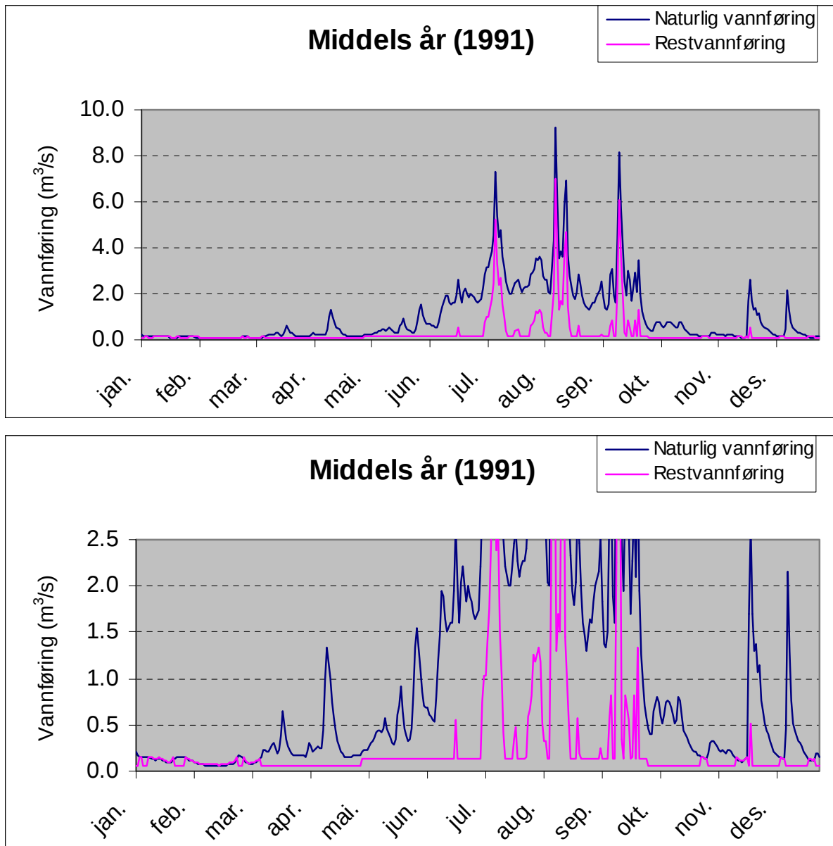
Figur 9.2 Plott som viser vassføringsvariasjonar Mundalselvi i eit middels (1991) år (før og etter utbygging). 18
