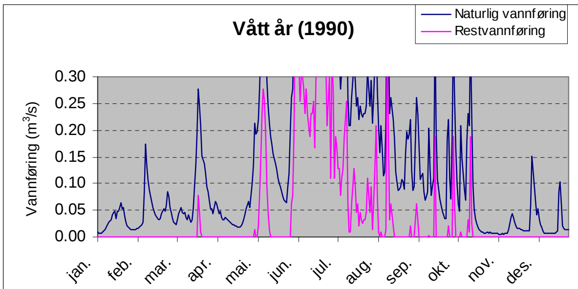
Figur 10.1 Plott som viser vassføringsvariasjonar i Botnagrovi i eit vått (1990) år (før og etter utbygging). 19
