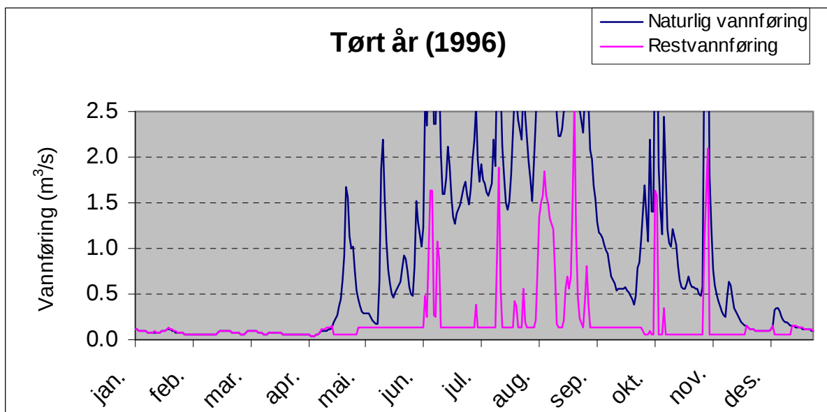
Figur 7.2 Plott som viser vassføringsvariasjonar i Mundalselvi i eit turt (1996) år (før og etter utbygging). 16
