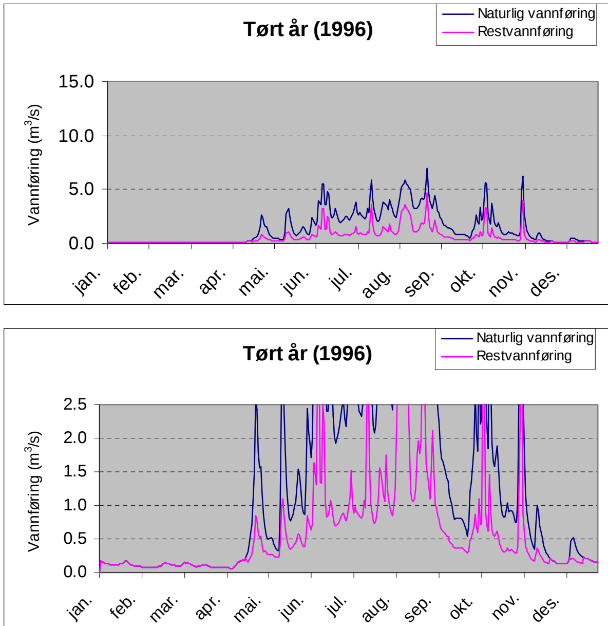
Figur 15. Restvannføringen i Mundalselvi rett oppstrøms kraftverket i et tørt år (1996) med en årsavrenning på 1,43 m 3 /s.
