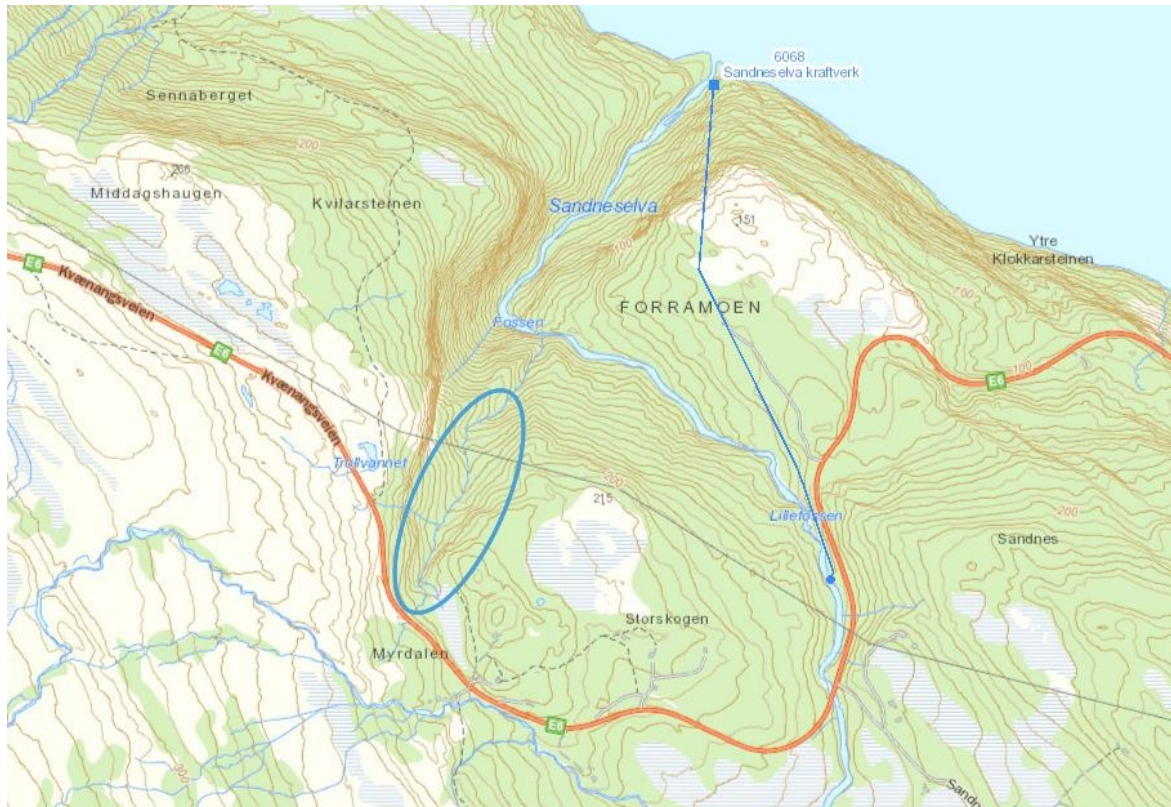
Figur 1. Sandneselva med planlagt inntak, vannvei og kraftstasjon for Sandneselva kraftverk. Aktuelt deponiområde i Myrdalen er markert med blå ellipse.
