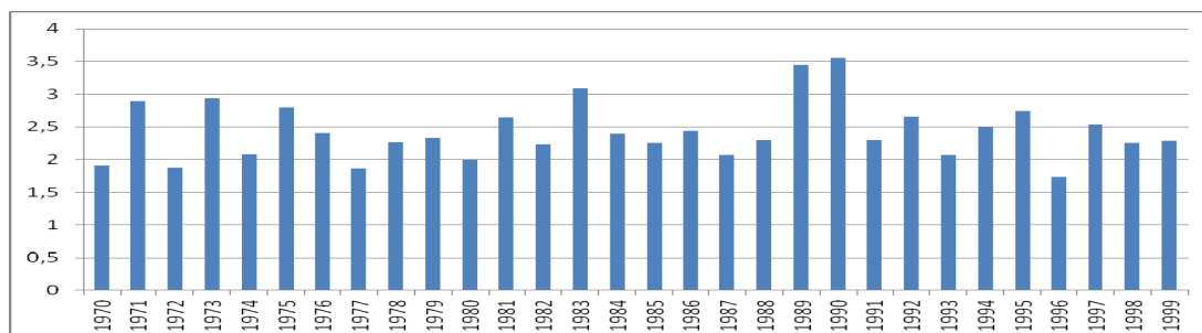
Diagram som viser variasjon i vassføring frå år til år (m 3 /s)
