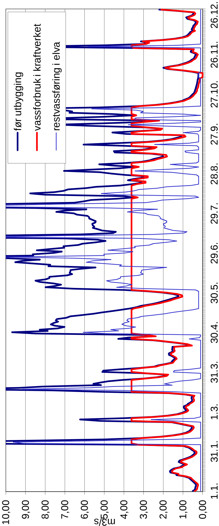
Vassføring før og etter utbygging i eit vått år (1990)
