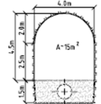
TVERSNITT B-B AV RØRTUNNEL 1:100
