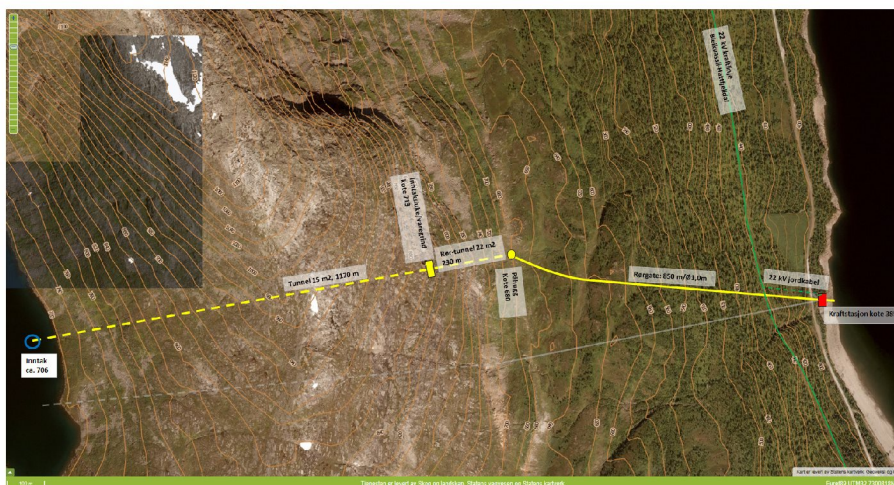
Figur 3-3 Stikkelvika kraftverk med justert planløsning (gul) og konsesjonssøkt trase (grå) Grunnlag: www.norgebilder.no
