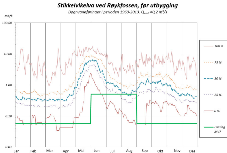
Figur: Naturlige vannføringer i Røykfossen i perioden 1969-2013 sammen med forslått minstevannføring, 500 og 57 liter/sekund (Etter vannmerke Glugvatn. Merk at y-aksen er logaritmisk).
