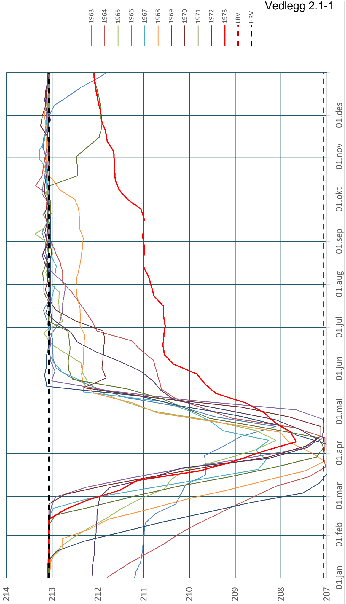
Vannstand Samsjøen 1963-1973 HRV = 213,07 LRV = 207,07
