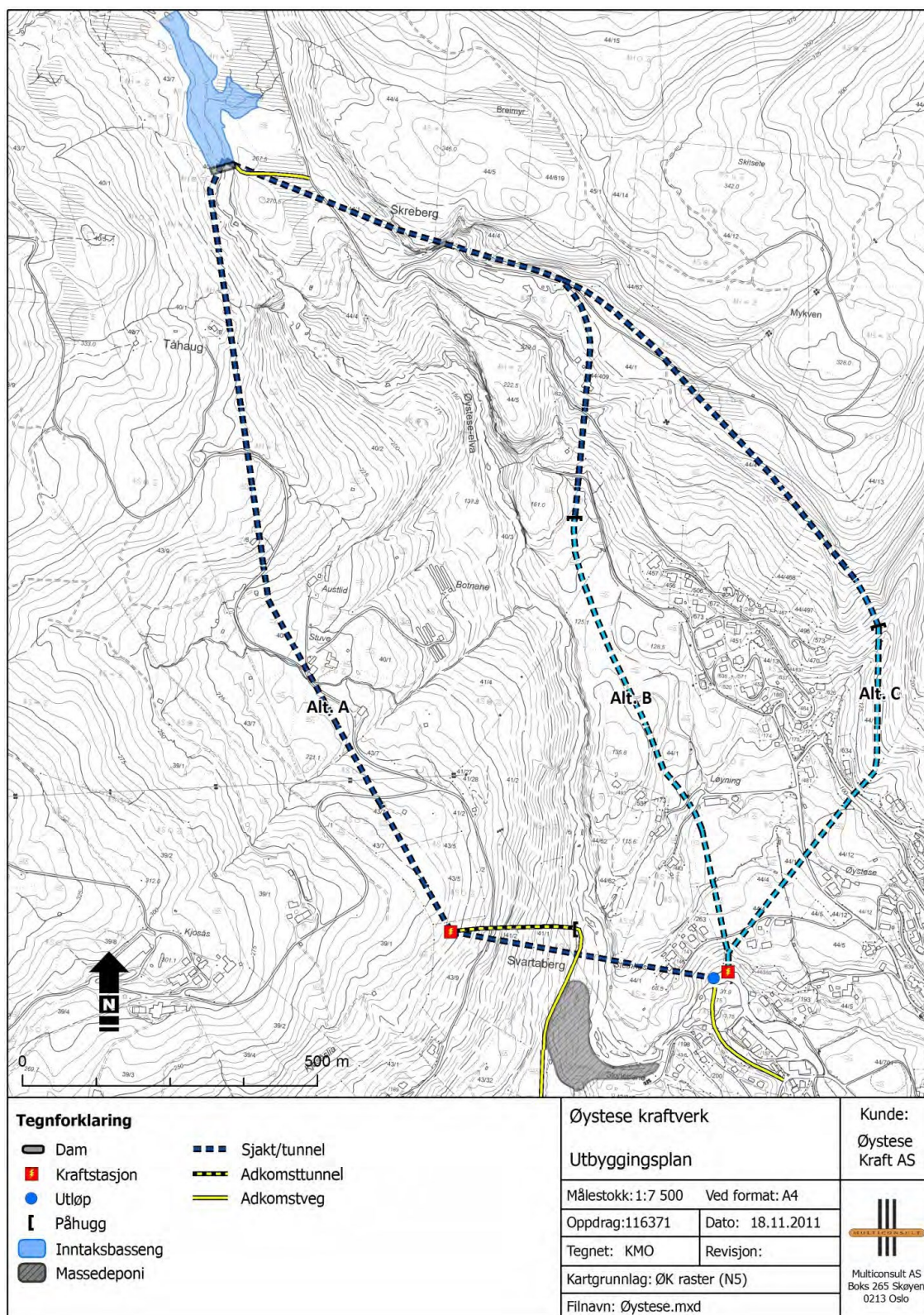
Figur 2: Kart over tiltaksområdet for Øystese kraftverk.
