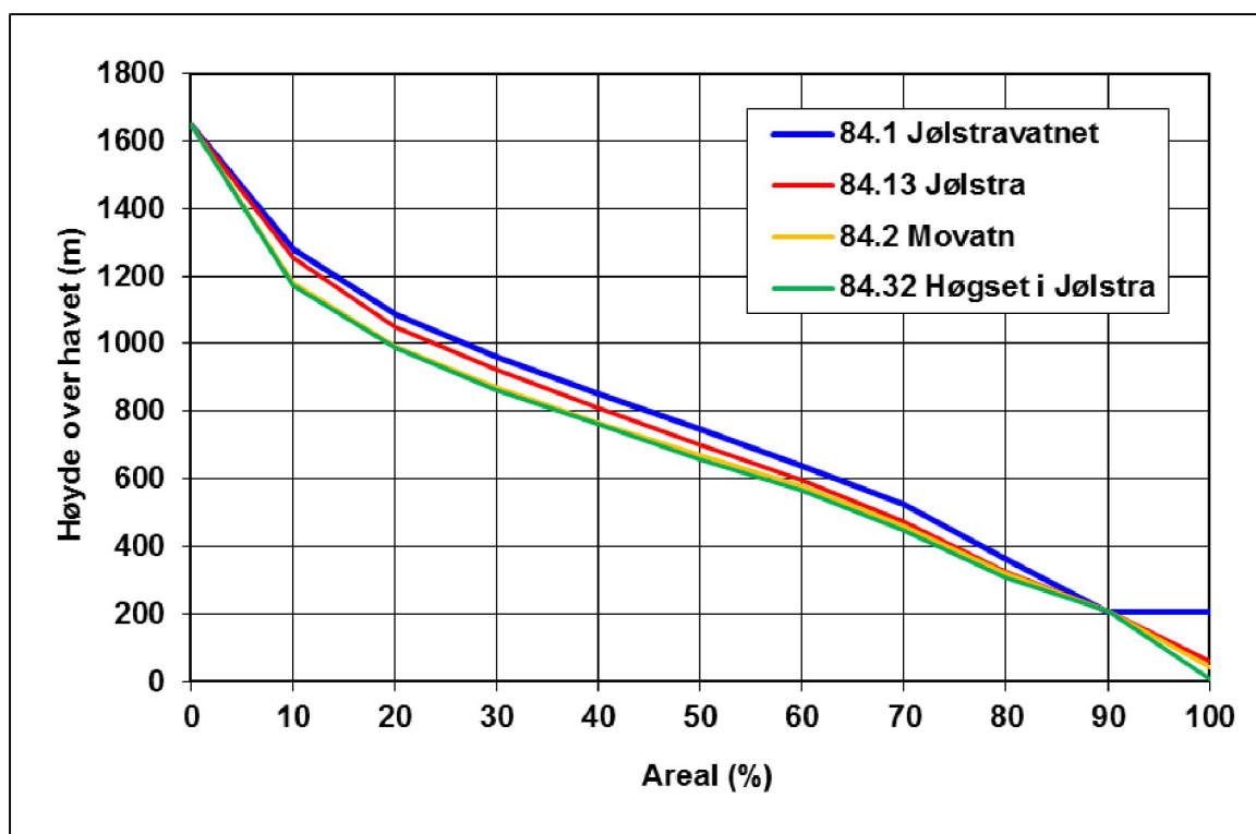
Figur 2. Hypsografiske kurver for totalfelt til målestasjoner.
