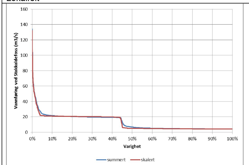
Figur 34. Sammenligning av varighetskurver til sommert og skalert vannføringsserie.
