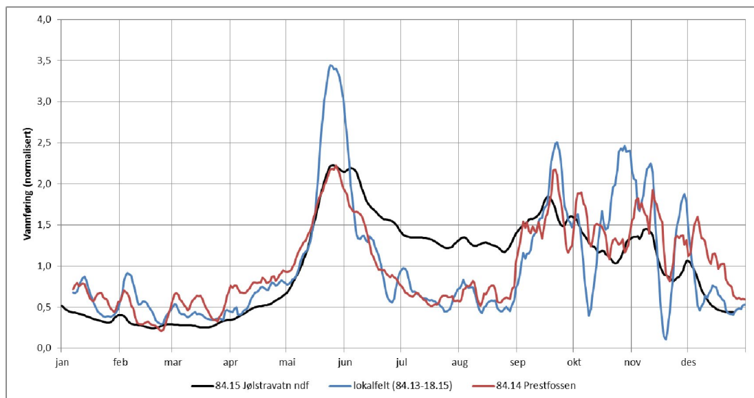
Figur 12 Midlere sesongvariasjon 1976-1986 (unntatt 1983) - glidende 7-døgnsmidler.
