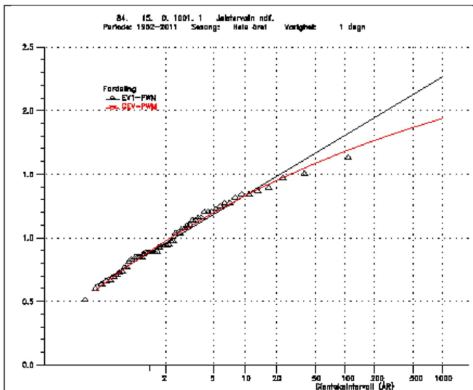
Figur 25. Flomfrekvensanalyse.
