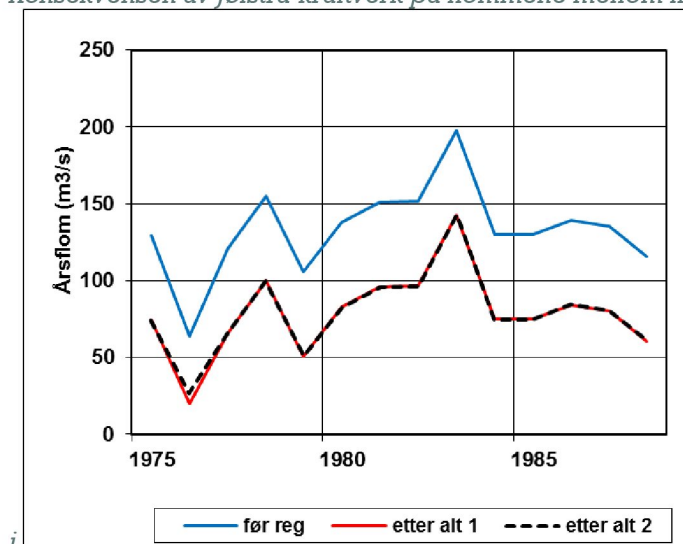
Figur 24. Middelflommen reduseres fra 133 til 79 m³/s og den største observerte flommen i perioden 1976-1988 fra 198 til 143 m³/s. Begge reduksjonene tilsvarer kraftverkets slukeevne på 55 m³/s.
