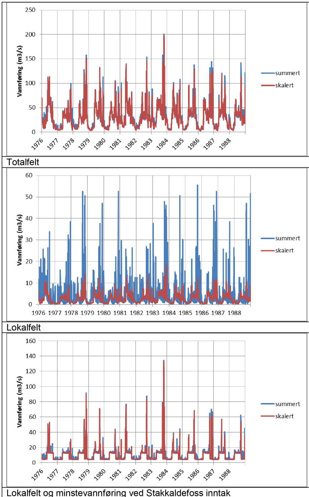
Figur 33. Sammenligning av sommert og skalert vannføringsserie.
