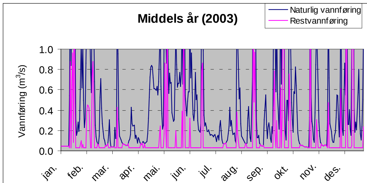
Figur 3 Plott som viser vassføringsvariasjonar i eit middels (2003) år (før og etter utbygging) iii
