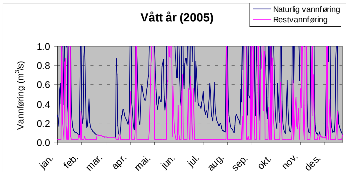
Figur 4 Plott som viser vassføringsvariasjonar i eit vått (2005) år (før og etter utbygging) iv
