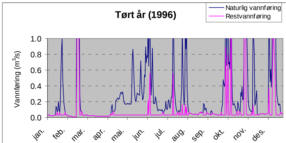
Figur 2 Plott som viser vassføringsvariasjonar i eit tørt (1996) år (før og etter utbygging) ii
