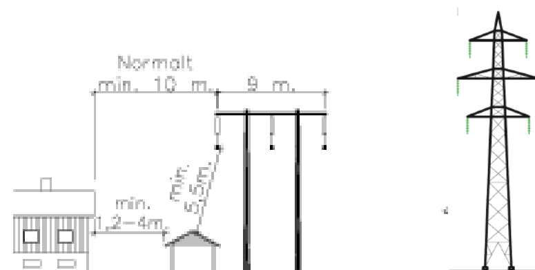
Figur 5.1. Figuren viser en 132 kV trestolpeledning til venstre og en 132 kV dobbeltkurs stålmast til høyre. Normalt bygge og ryddebelt for denne typen ledninger er ca. 29 meter for masten til venstre og ca. 28 meter for dobbeltkursmasten til høyre.
