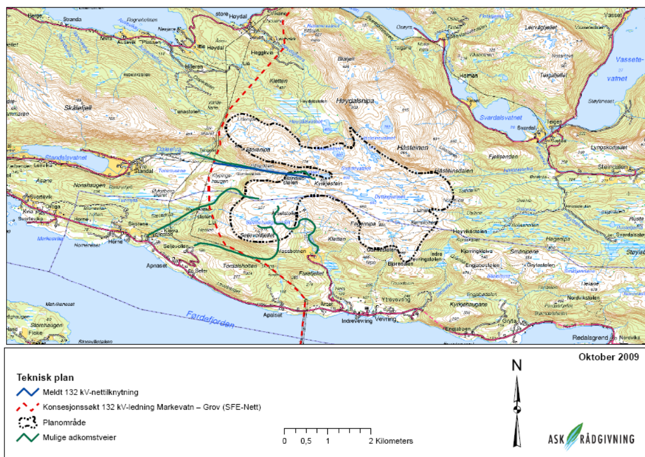
Figur 5.2. Nettløsning for Kyrkjestein vindkraftanlegg
