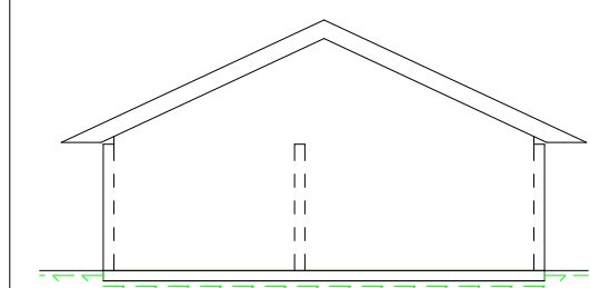
SNITT 3-3 1 : 100
