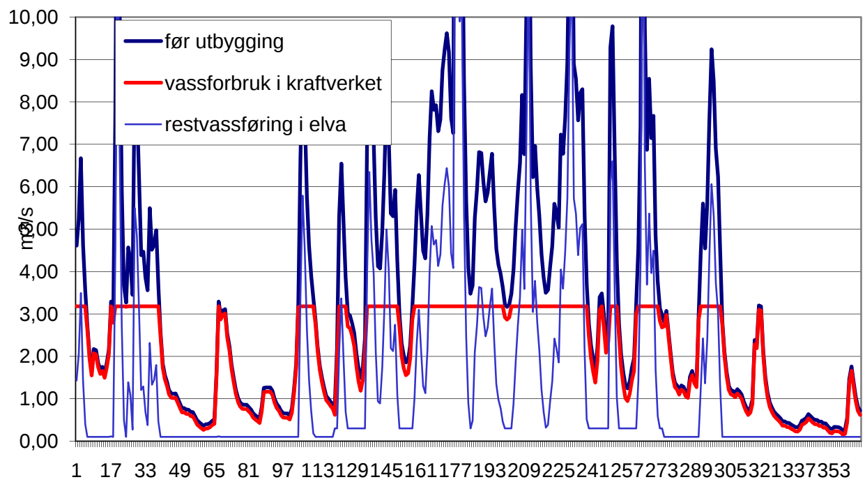
Figur 4. Plott som viser vannføringsvariasjoner i et vått (1989) år (før og etter utbygging).
