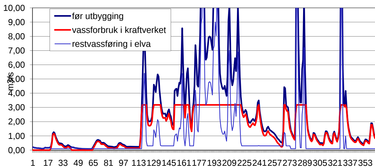
Figur 3. Plott som viser vannføringsvariasjoner i et middels (1994) år (før og etter utbygging).
