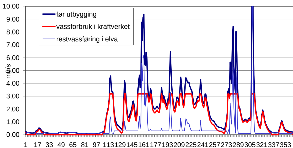
Figur 2. Plott som viser vannføringsvariasjoner i et tørt (1996) år (før og etter utbygging).
