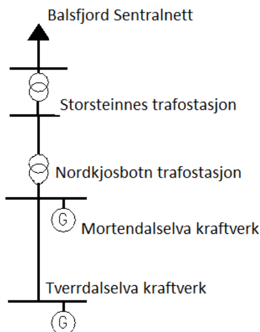
Figur 2 Enlinjeskjema for avgang fra Nordkjosbotn Trafostasjon
