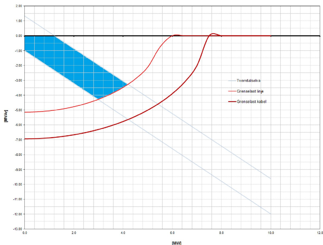
Figur 1 Krav til reguleringsområde som funksjon av aktiv produksjon ved Tverrdalselva i Storfford kommune
