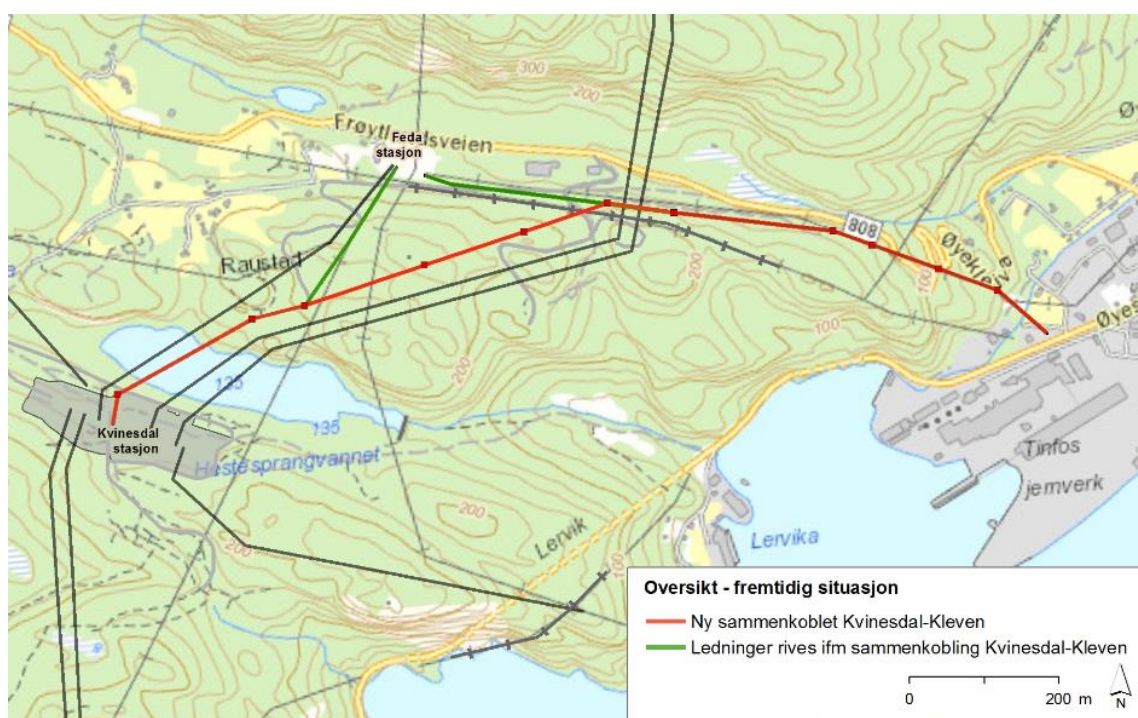
Figur 2: Rød strek viser ny ledning mellom Kvinesdal og Kleven. Grønn strek viser ledninger som skal rivet etter at Kvinesdal og Kleven ledningen er sammenkoblet.
