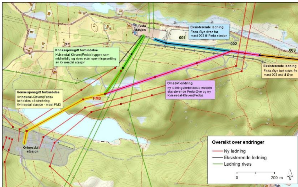
Figur 1: Ny ledning er vist med rosa strek mellom mast 003 og FM3. Ledning som skal rives er vist med grønn strek.
