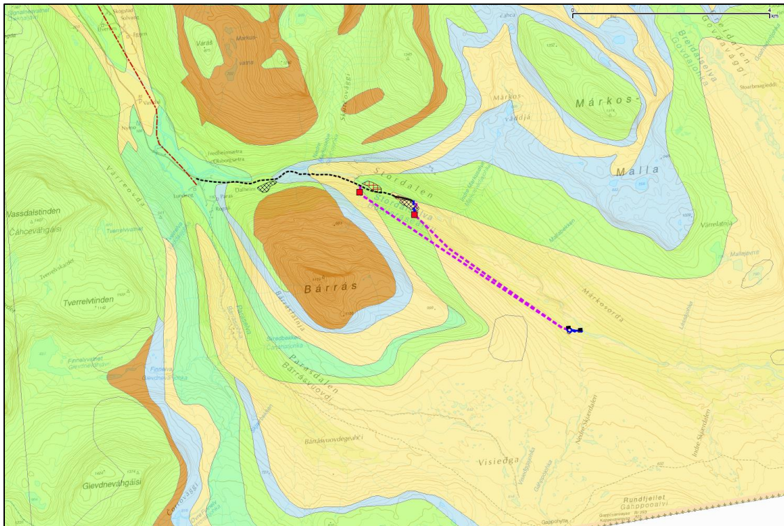
Figur 10. Berggrunnskart over området rundt Stordalen. Rundt kraftverksområdet er det metagråvakke (grønn farge) mens det et stykke oppstrøms kommer inn en stor formasjon med metaarkose (gul farge). Blå farge viser karbonatbergarter, oftest marmor, mens brun farge er amfibolitt og andre mafiske bergarter. Kilde: Norges geologiske undersøkelse.
