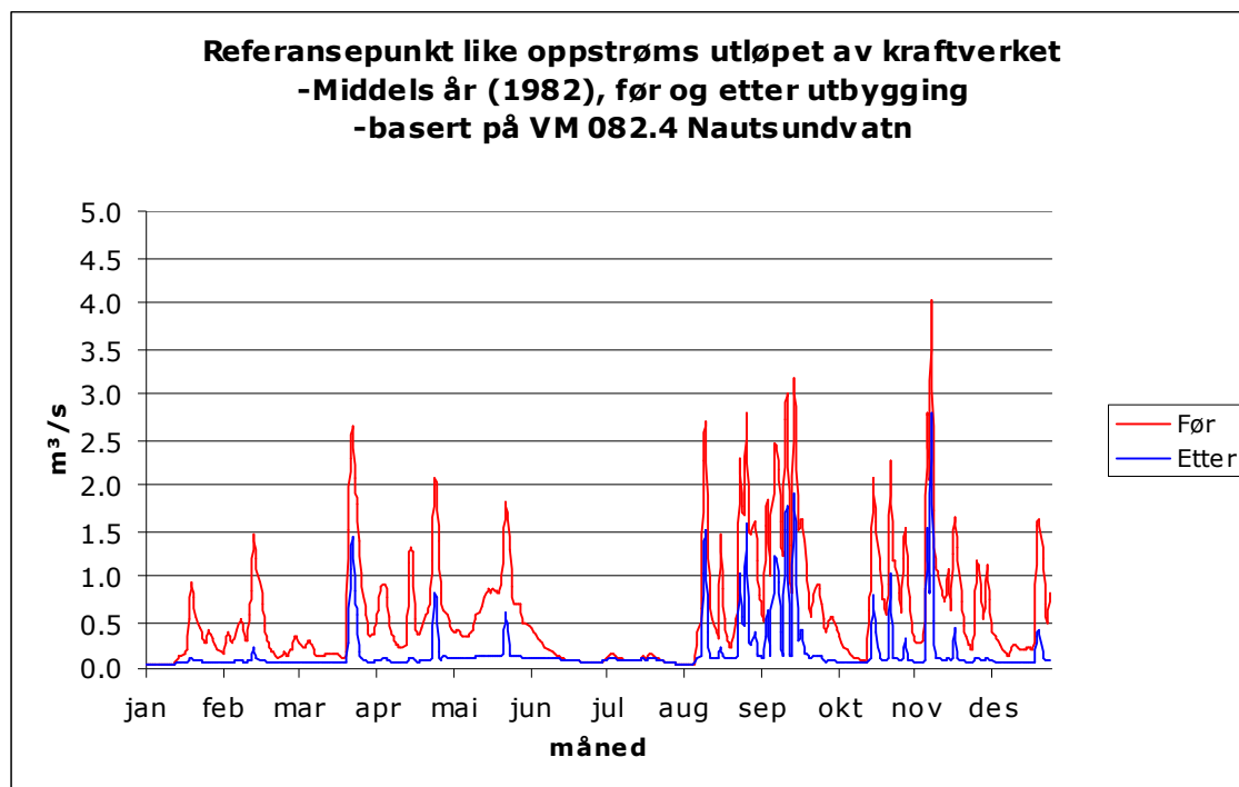
Fig. 13: Plott av vassføringsvariasjonar i eit middels år (1982) før og etter utbygging Stordalsvatn.
