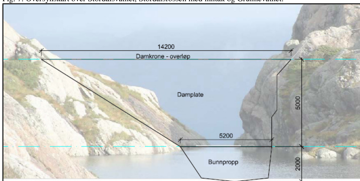
Fig. 8: Prinsippsskisse for inntaksdam sett oppstrøms.
