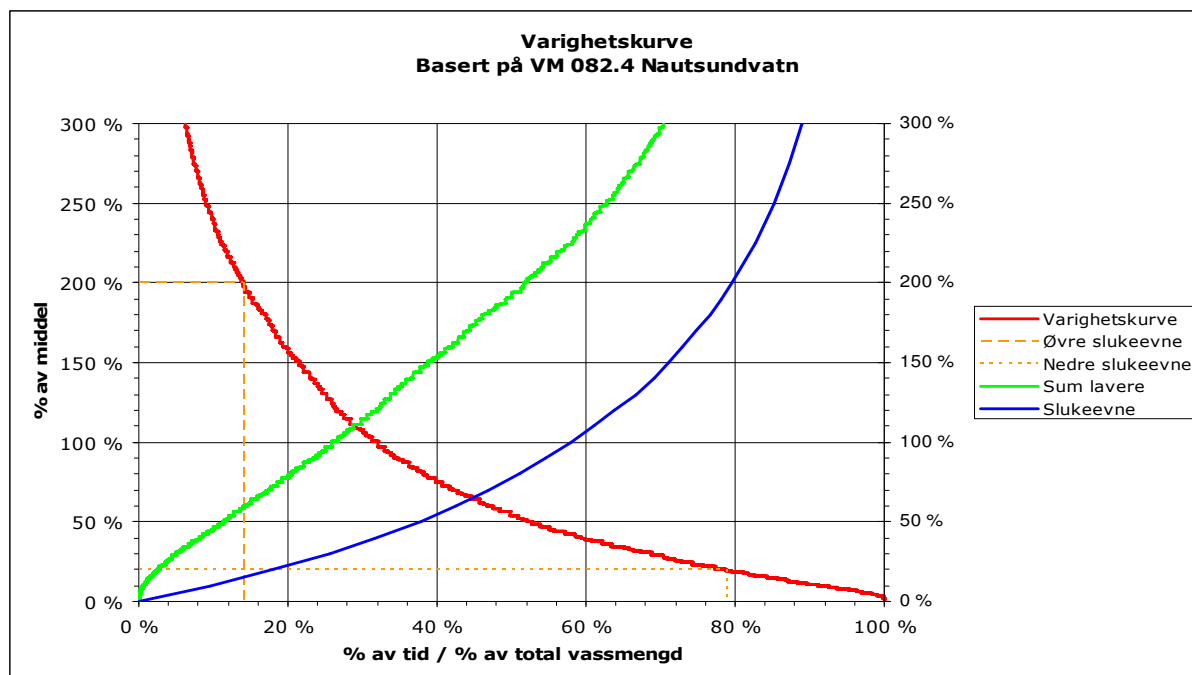
Fig. 5: Varighetskurve Stordalsvatnet kraftverk basert på vassmerke Nautsundvatn.
