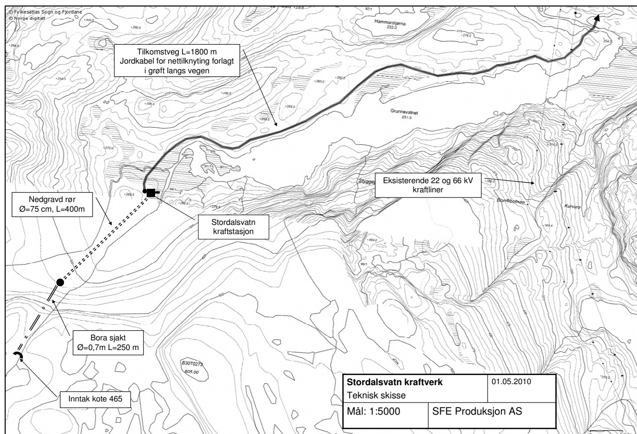
Fig. 6: Teknisk skisse Stordalsvatn kraftverk.
