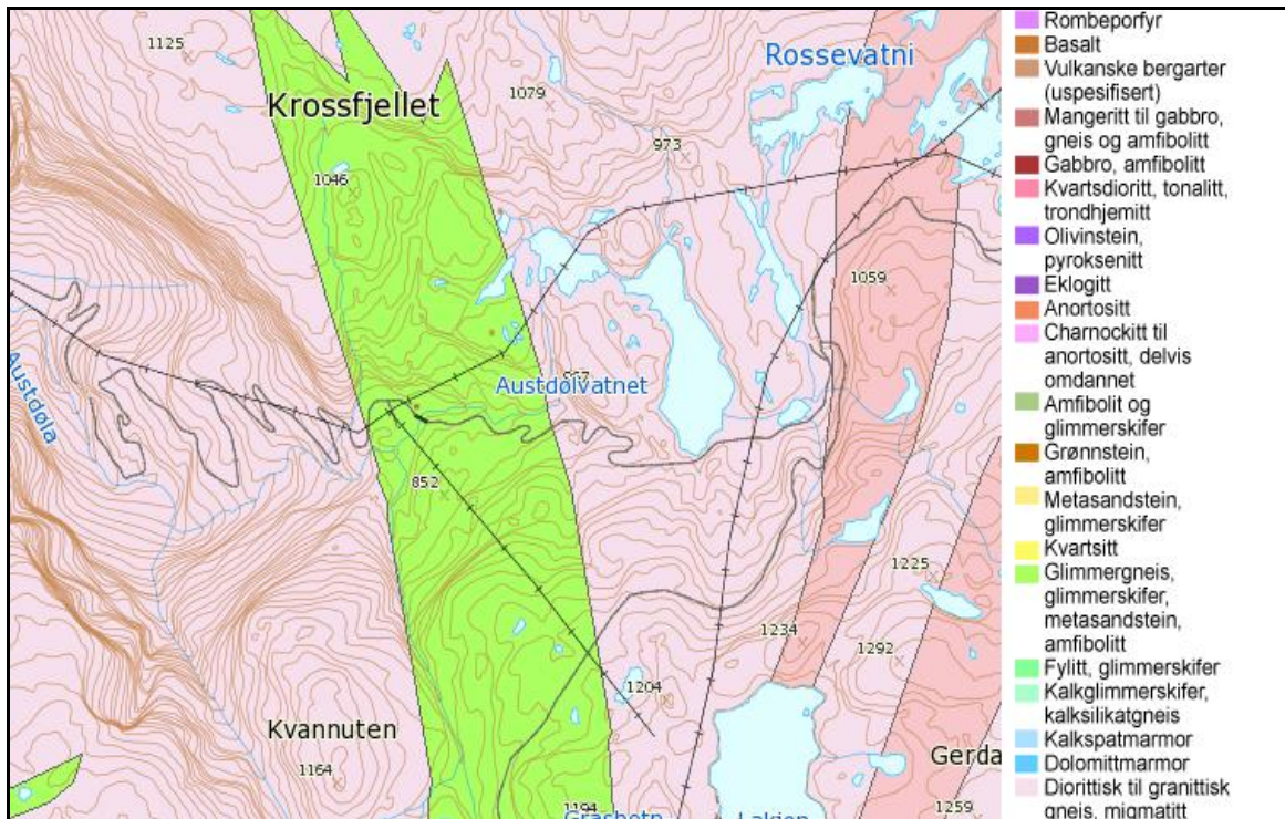
Figur 5. I henhold til NGUs berggrunnskart består berggrunnen av diorittisk til granittisk gneis, migmatitt. Kilde: Norges geologiske undersøkelse.
