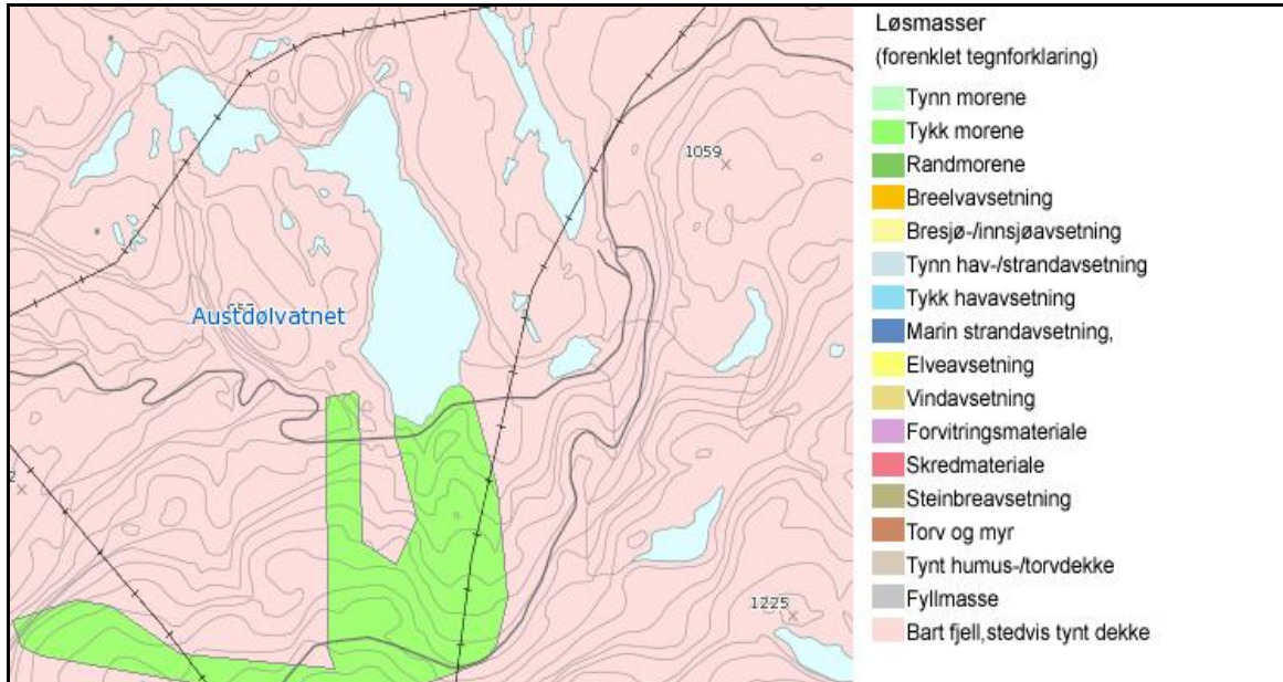
Figur 6. NGU's løsmassekart viser at influensområdet domineres av bart fjell, med mindre innslag tykk morene. Kilde: Norges geologiske undersøkelse.
