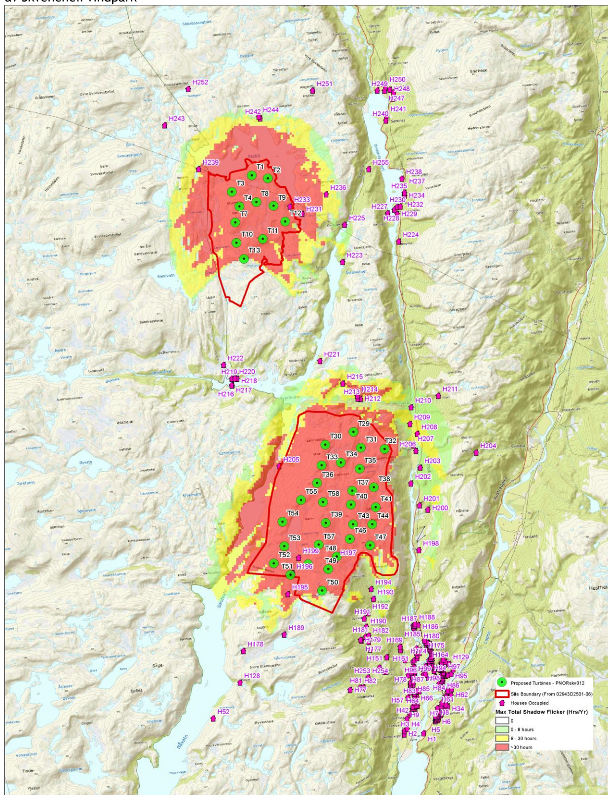
Figur 4.1: Skyggekart som viser total teoretisk årlig skyggekastvarighet for hver eiendom som følge av Skvенеheii vindpark
