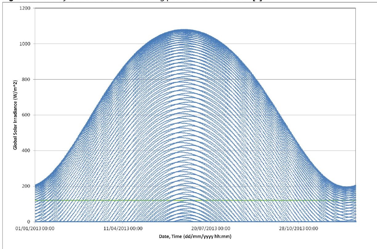
Figur 5.1: Variasjon i teoretisk solinnstråling på Skveneheii i år 2013 [7].
