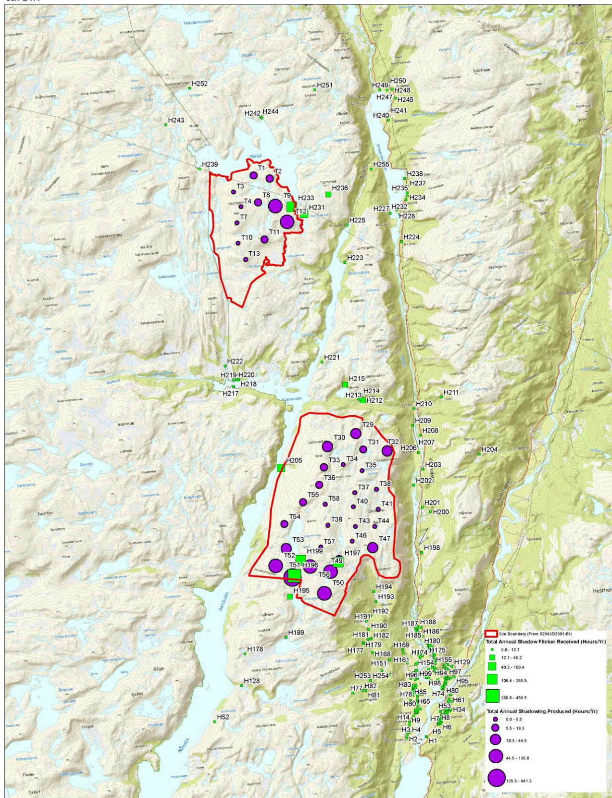
Figur 4.3: Teoretisk maksimalt årlig skyggekast for hver eiendom og varighet forårsaket av hver turbin
