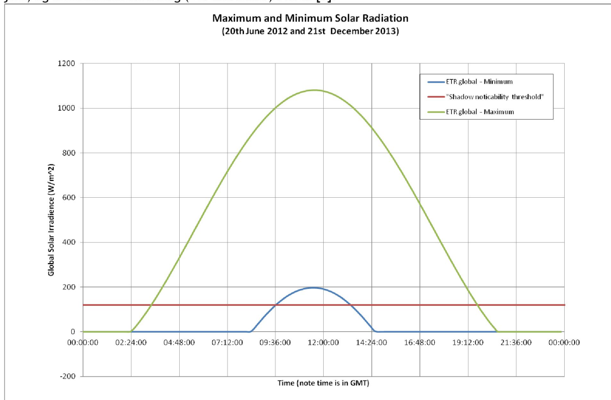
Figur 5.2: Variasjon i teoretisk solinnstråling på Skveneheii på dagen for maksimal solinnstråling (20. juni) og minimal solinnstråling (21. desember) i 2013 [7].
