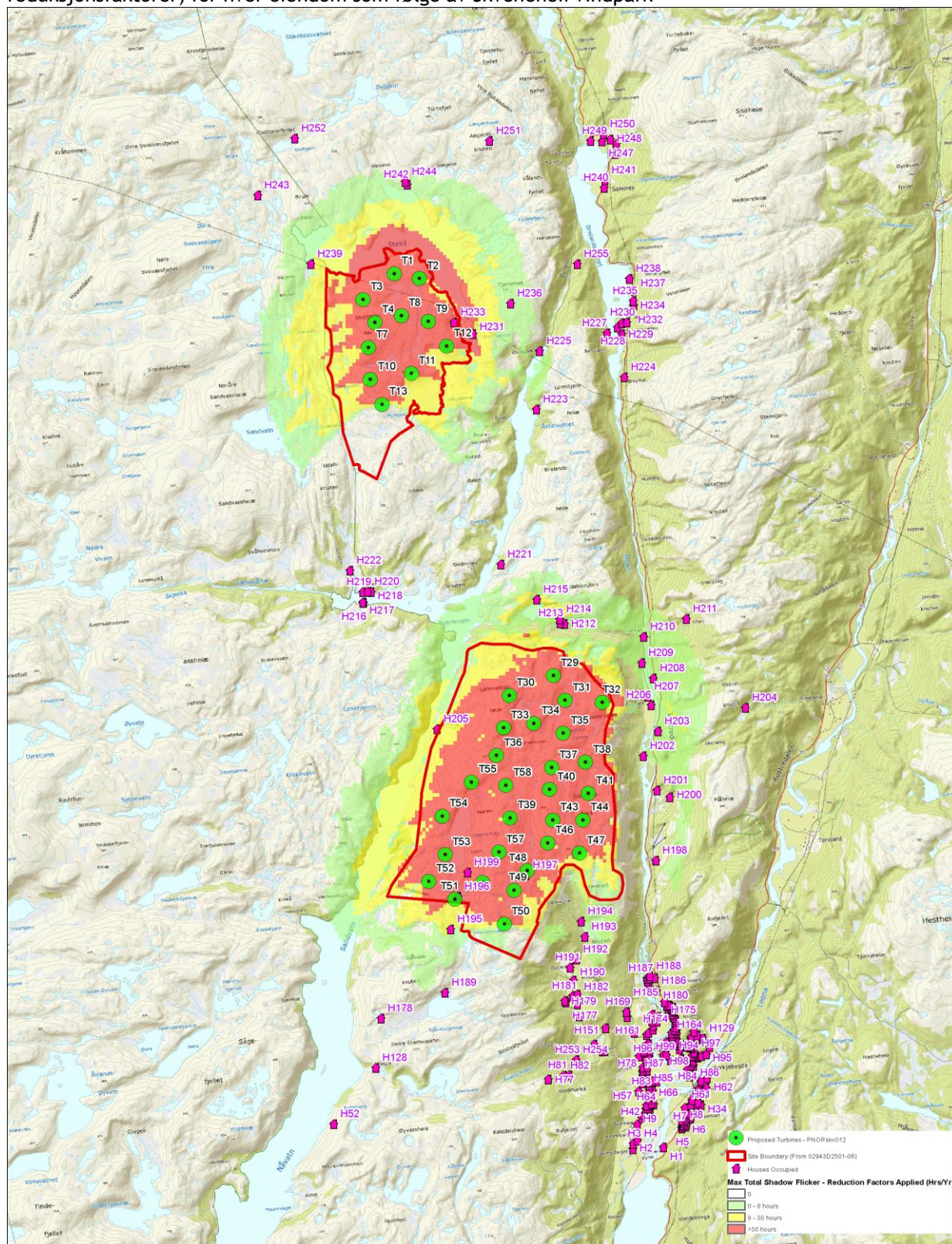
Figur 4.4: Skyggekart som viser total resulterende årlig skyggekastvarighet (med reduksjonsfaktorer) for hver eiendom som følge av Skvенеhei vindpark
