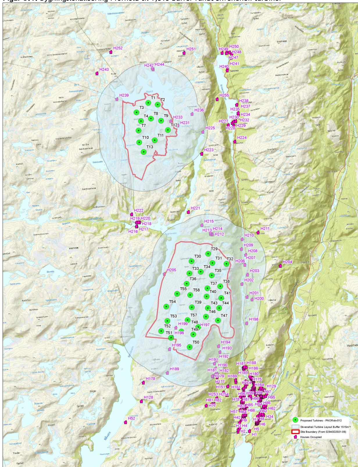
Figur 3.1: Bygningslokalisering i forhold til 1,515 buffer rundt Skvenehei turbiner
