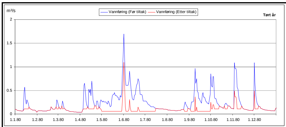
Figur 6. Plott som viser vannføringsvariasjoner i et tørt (1980) år (før og etter utbygging). 16
