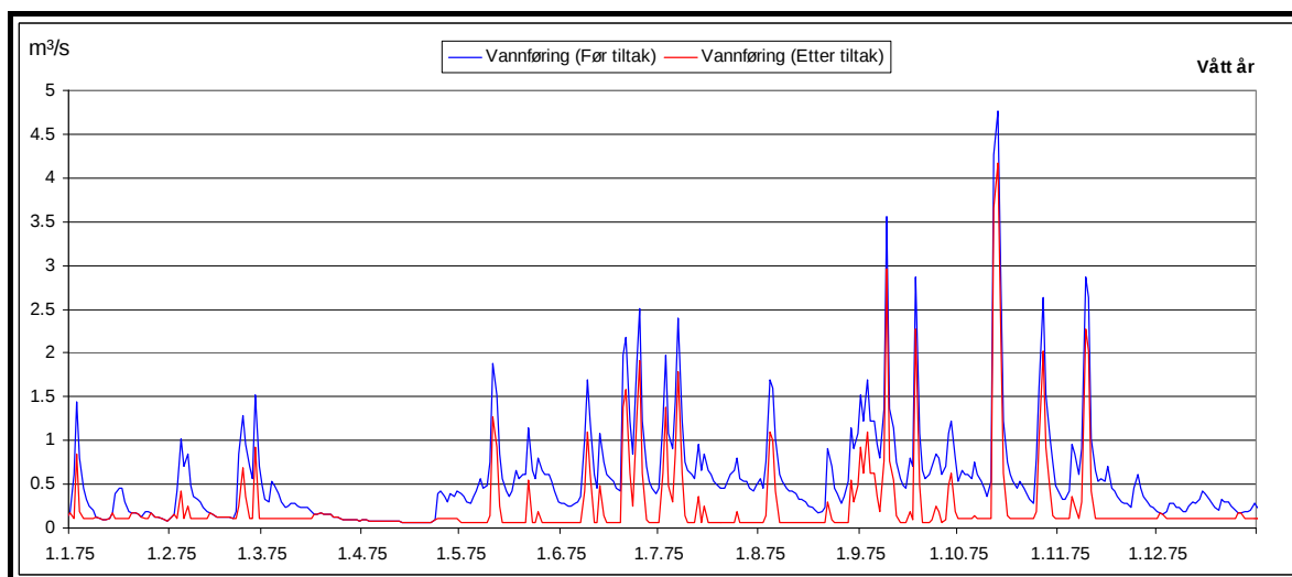
Figur 8. Plott som viser vannføringsvariasjoner i et vått (1975) år (før og etter utbygging). 18
