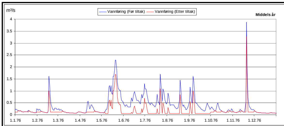
Figur 7. Plott som viser vannføringsvariasjoner i et middels (1976) år (før og etter utbygging). 17
