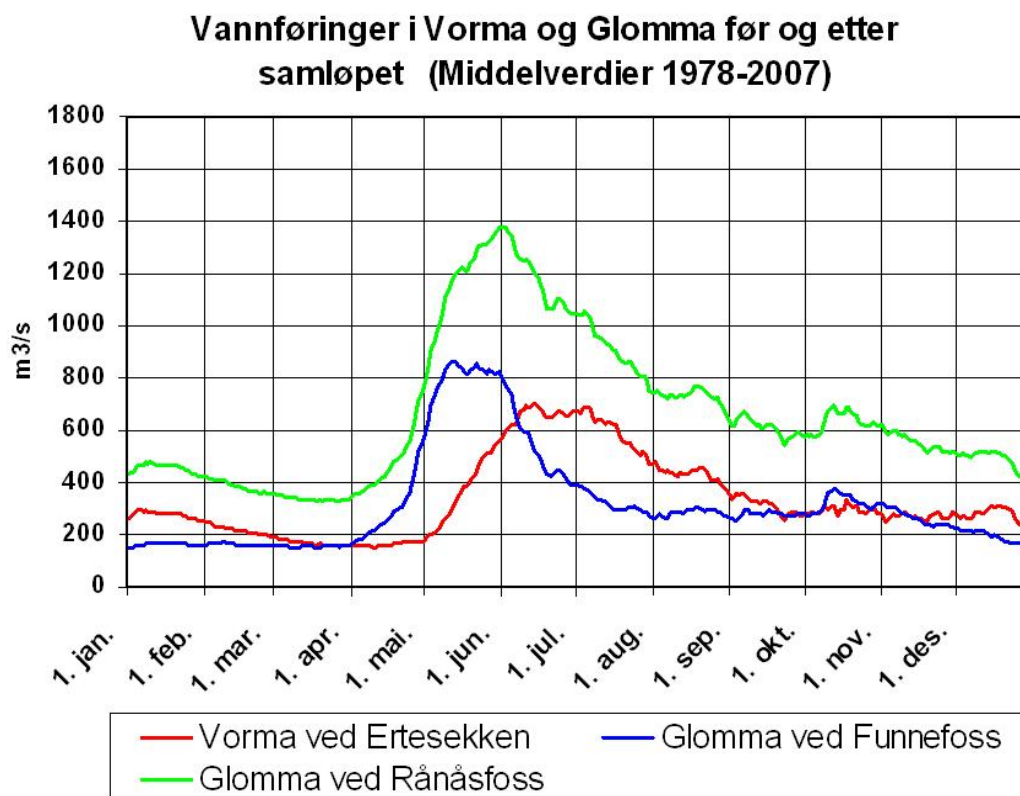
Figur 1. Vannføringskurve for Vorma ved Ertesekken, Glomma ved Funnefoss og Glomma ved Rånåsfoss basert på middelverdier i perioden 1978-2007.
