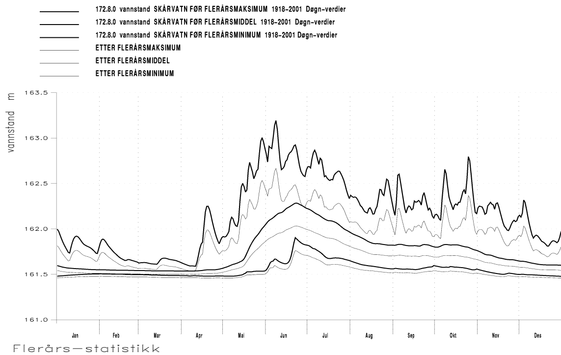
Figur 5.2.3 : Vannstander i Skárvatn før og etter overføring av Røvatn til Hjertvatn magasin.
