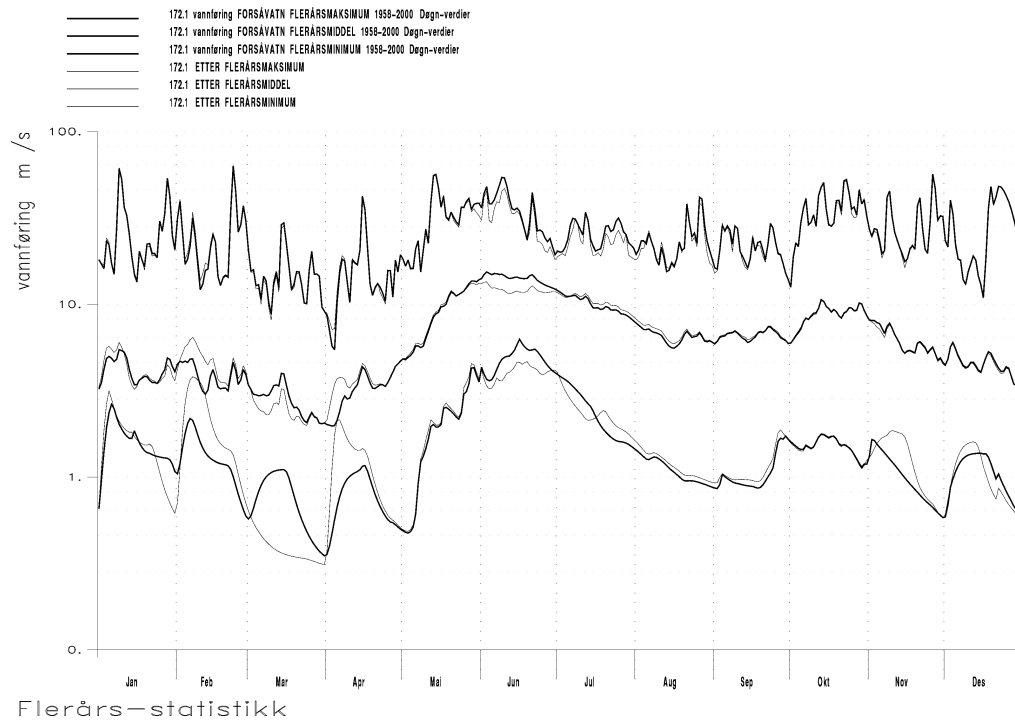
Figur 5.7.a: Vannføringer i elva ut av Forsåvatn før og etter overføring av Røvatn til Hjertvatn magasin.
