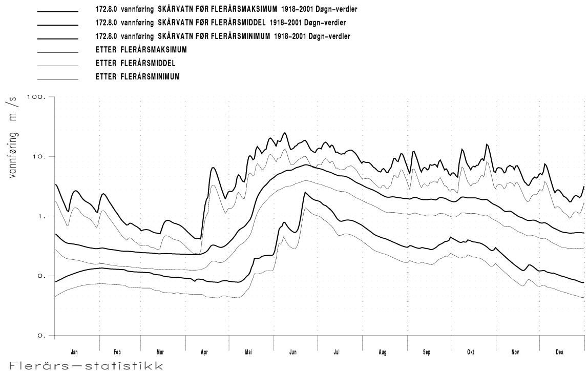
Figur 5.2.2: Vannføringer i elva ut av Skårvatn før og etter overføring av Røvatn til Hjørtvatn magasin. Merk logaritmisk vannføringsskala., laveste hovedstrek er 10 l/s neste er 100 l/s osv.
