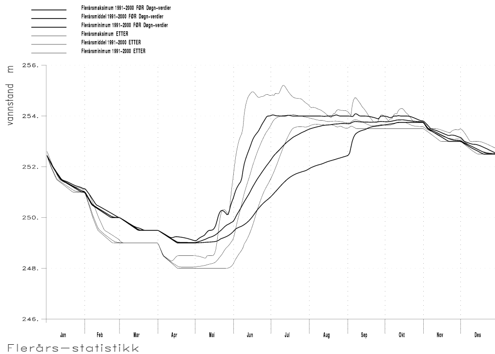
Flerårs-statistikk Figur 5.5.2: Simulerte vannstander i Hjertvatn for perioden 1991 - 2000 før og etter overføring av Røvatn til Hjertvatn magasin og økning av innstallasjonen i kraftverket.
