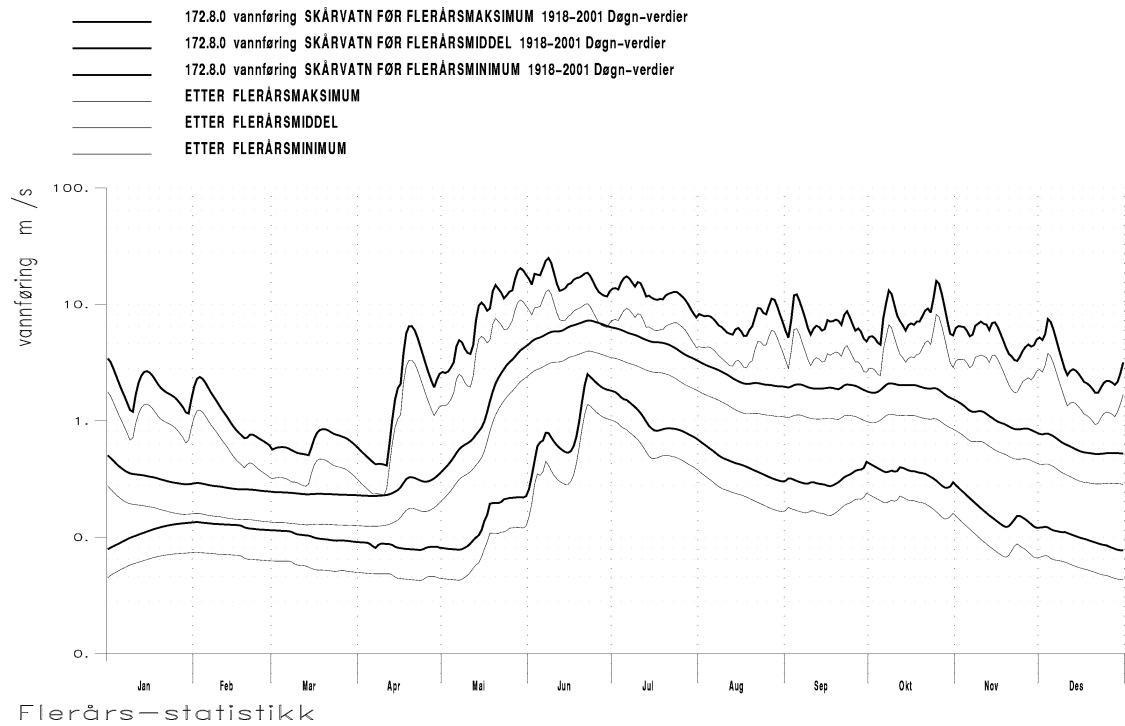
Figur 5.3.1: Vannføringer i elva ut av Melkevatn før og etter overføring av Røvatn til Hjertvatn magasin.
