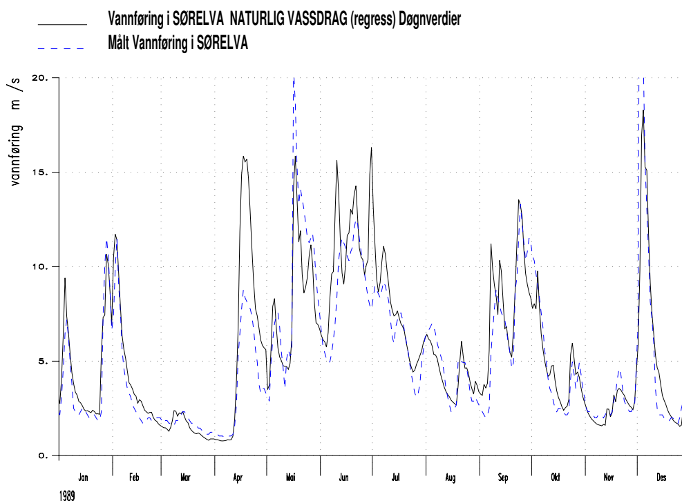
Figur 5.6.2.c: Vannføringer i Sørelva før og etter Hjertvatn kraftverk. Daglige vannføringer i et vått år 1989.
