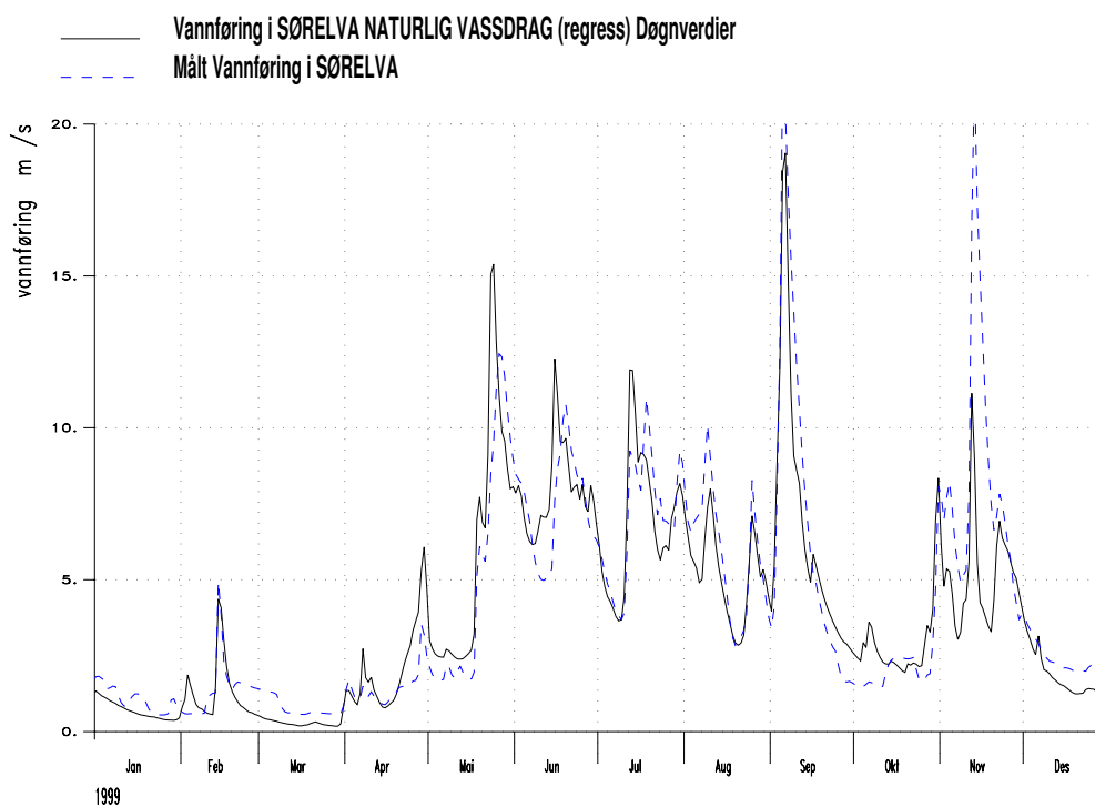
Figur 5.6.2.b: Vannføringer i Sørelva før og etter Hjertvatn kraftverk. Daglige vannføringer i et normalår 1999.
