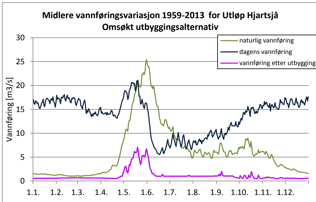
Figur 3-2. Årsprofil for middelvannføring nedenfor inntaket til Sauland 1: naturlig vannføring (før utbygging av Hjarthøla kraftverk), eksisterende vannføring (med Hjarthøla kraftverk) og vannføring etter utbygging av det konsesjonssøkte utbyggingsalternativet for Sauland kraftverk.
