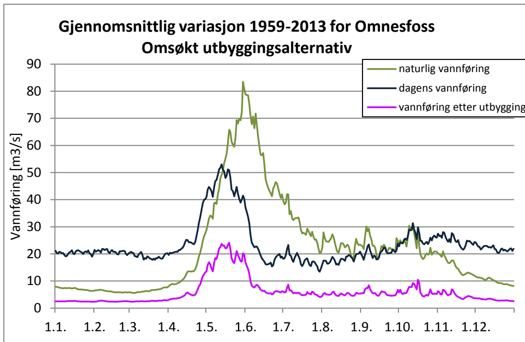
Figur 3-3. Årsprofil for middelvannføring ved Omnesfoss: naturlig vannføring (før utbygging av Hjarthøla kraftverk), eksisterende vannføring (med Hjarthøla kraftverk) og vannføring etter utbygging av det konsesjonssøkte utbyggingsalternativet for Sauland kraftverk.
