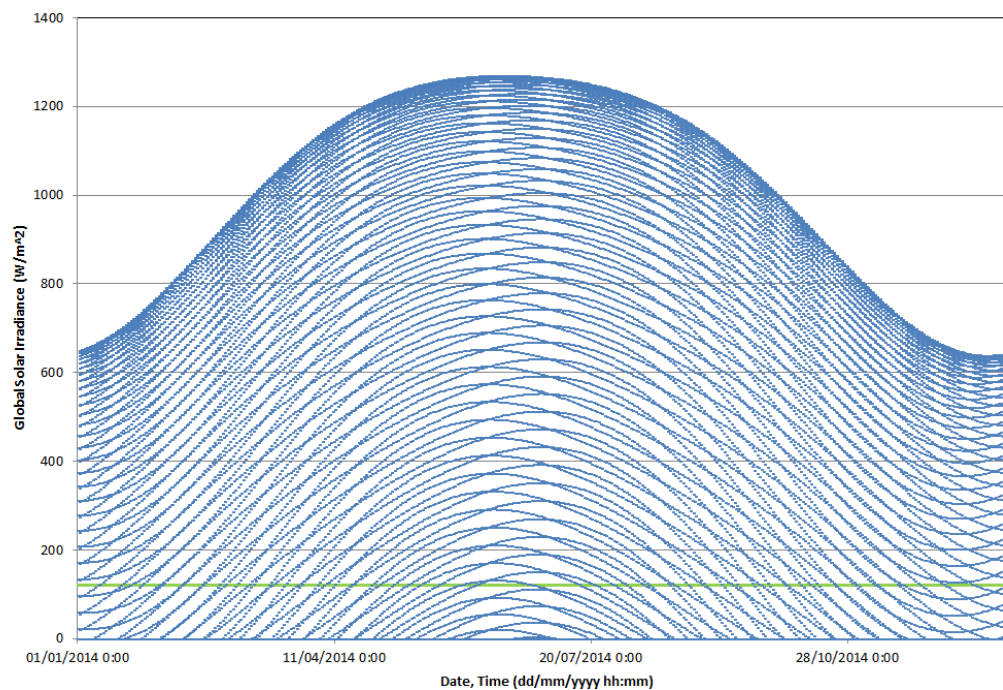
Figur 5.1: Variasjon i teoretisk solinnstråling på Hovatn Aust i år 2014 [6].
