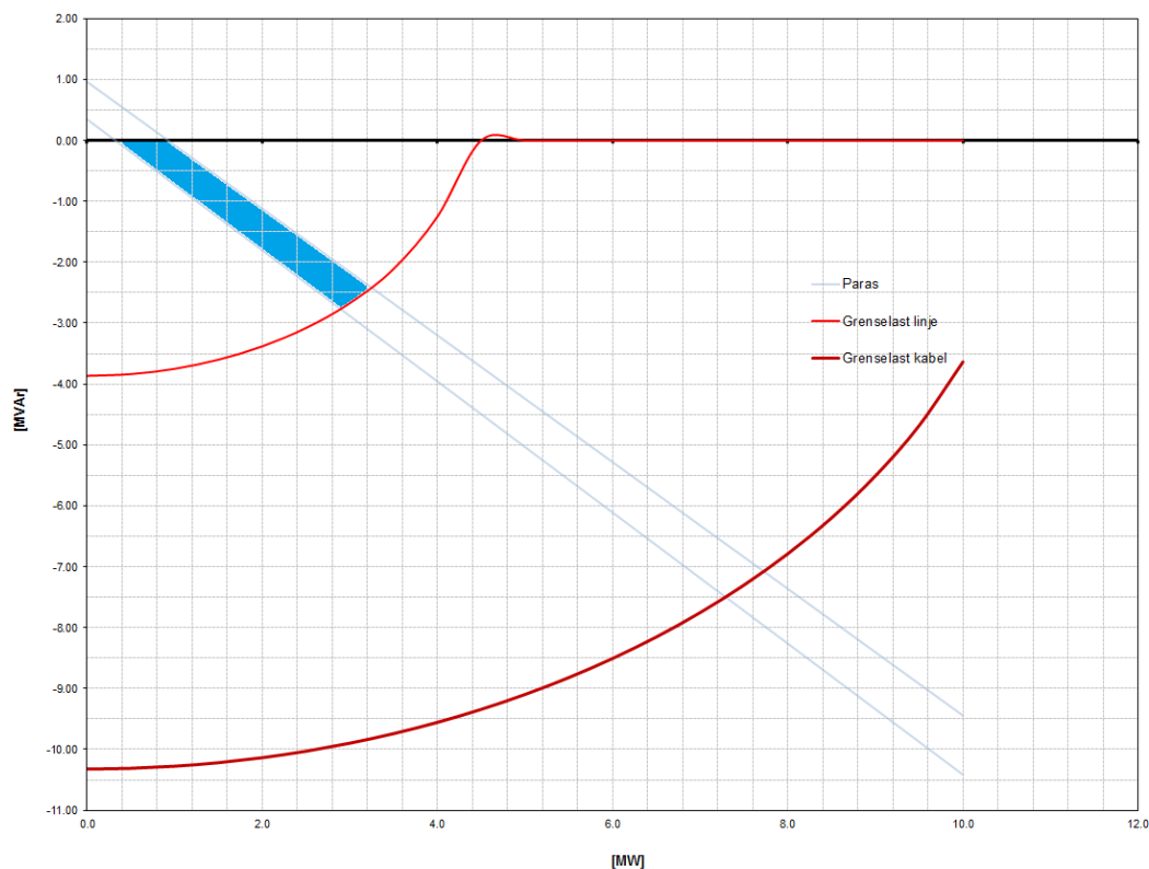
Figur 1 Krav til reguleringsområde som funksjon av aktiv produksjon ved Paras i Storfjord kommun
