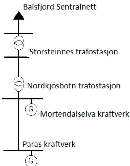
Figur 2 Enlinjeskjema for avgang fra Nordkjosbotn trafostasjon
