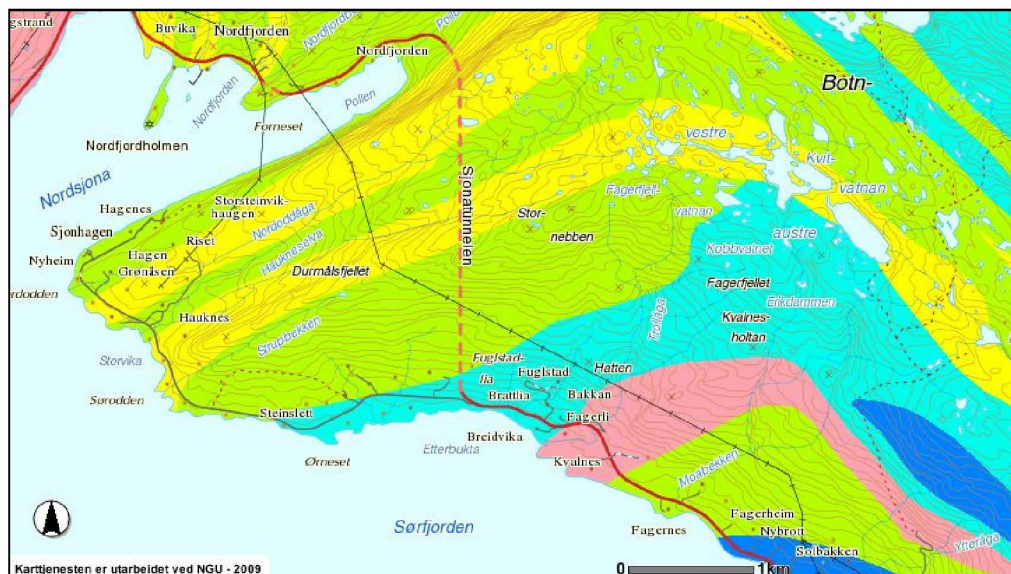
Figur 13. I henhold til NGU's berggrunnskart består berggrunnen i influensområdet av flere ulike bergarter. Kvitvatnan og området i nordvest består berggrunnen hovedsakelig av kvartitt (gul) og glimmergneis/glimmerskifer, metasediment og amfibolitt (grønn). Sør for Kvitvatnan ligger det et større felt med kalkglimmerskifer, kalksilikatgneis (lys blå). Moabekken renner gjennom diorittisk til granittisk gneis, migmatitt (rosa) og glimmergneis/glimmerskifer, metasediment og amfibolitt (grønn).
