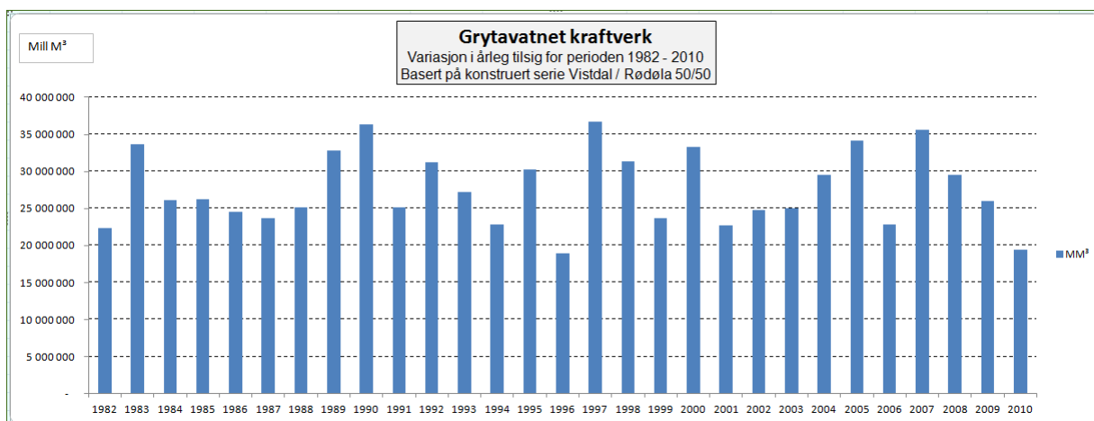
Figur 2.2.1.2 Variasjon i årleg tilsig til Grytuvatnet kraftverk 1982 – 2010.
