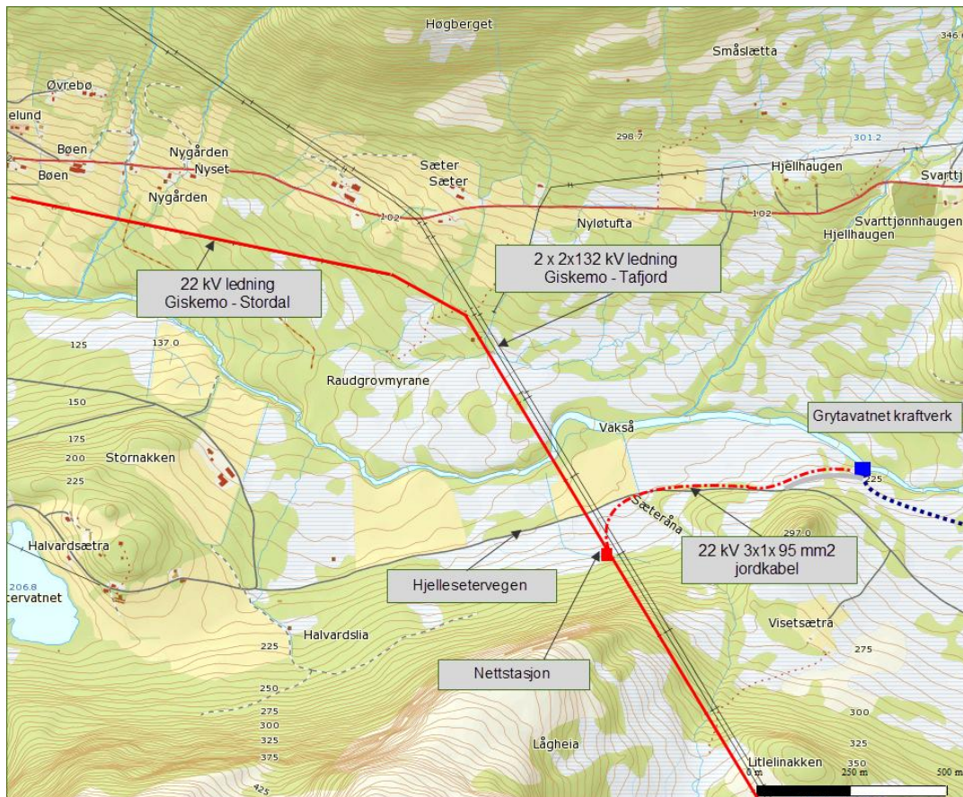
Figur 2.2.10.1 22 kV nettilknytning for Grytavatnet kraftverk
