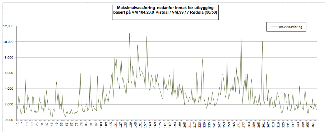
Figur 2.2.1.3. Maksimumsvassføring dag for dag perioden 1982 -2010 nedstrøms inntaket til Grytuvatnet kraftverk før utbygging.
