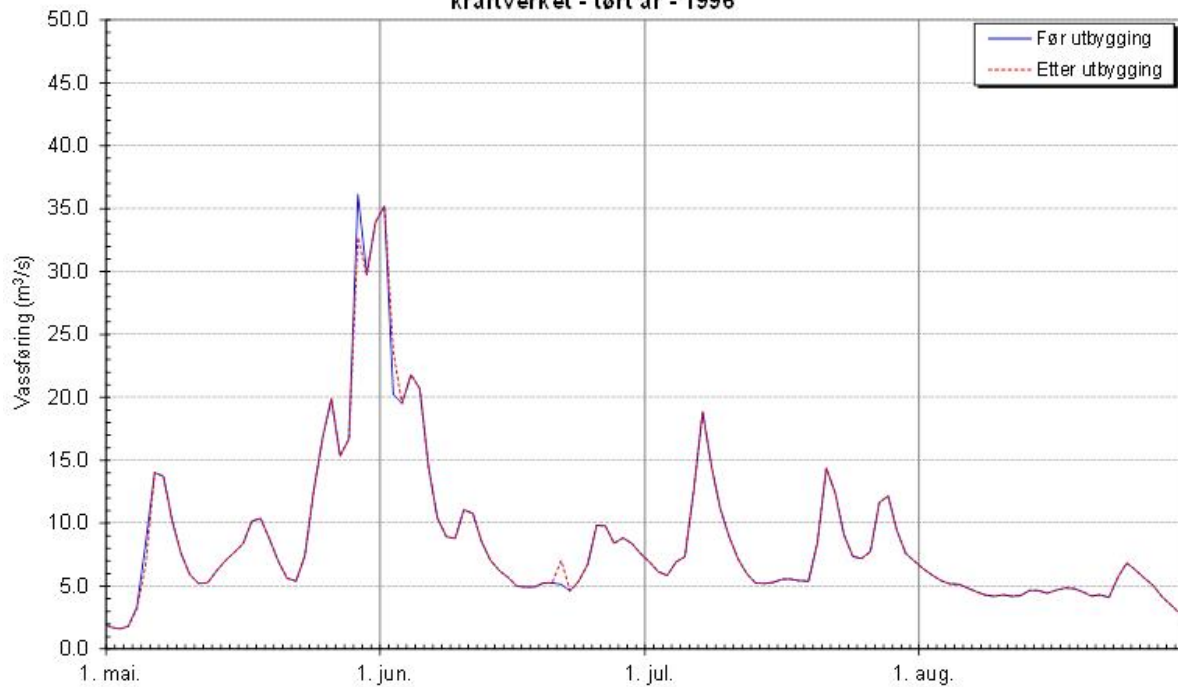
Gjengedal kraftverk. Uten reg av Storvatnet - Vassføring nedstrøms utløpet av kraftverket - tørt år - 1996
