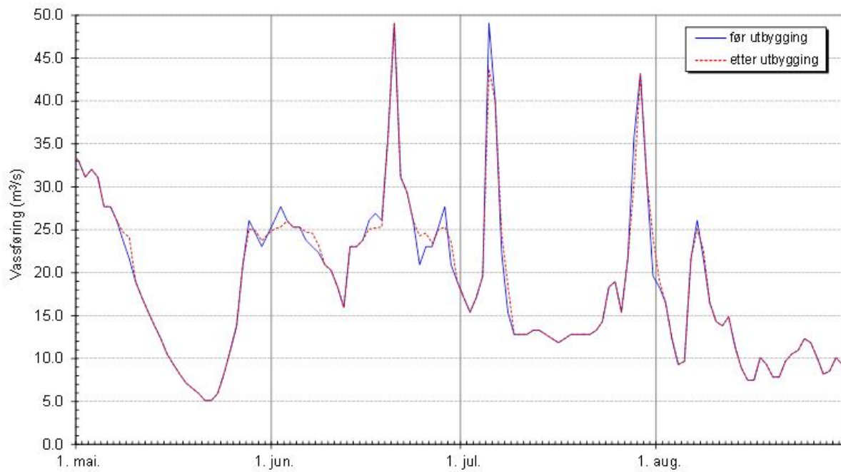
Gjengedal kraftverk. Uten reg av Storvatnet - Vassføring nedstrøms utløpet av kraftverket - vått år - 1990
