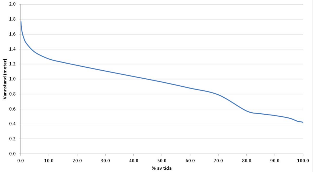
Varighetskurve for vannstand i Dalevatnet - måleperiode 02.06.2012 - 21.3.2014
