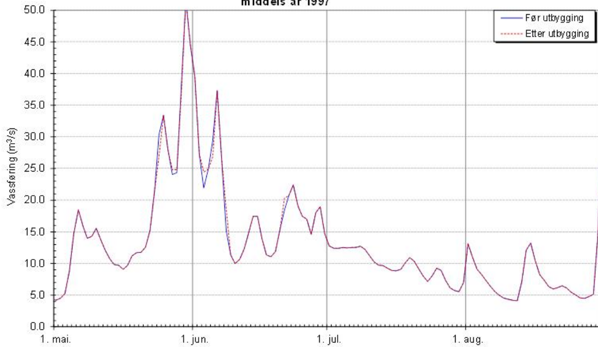
Gjengedal kraftverk. Uten reg av Storstvatnet - Vassføring nedanfor kraftverket - middels år 1997
