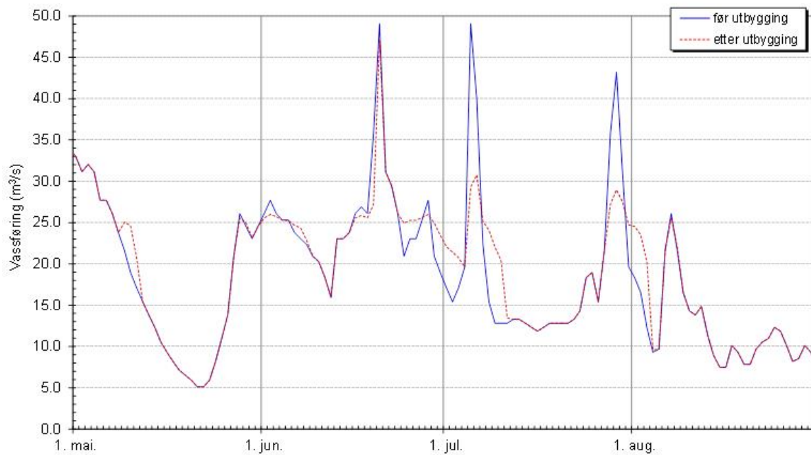
Gjengedal kraftverk. Med reg av Storevatnet - Vassføring nedstrøms utløpet av kraftverket - vått år - 1990
