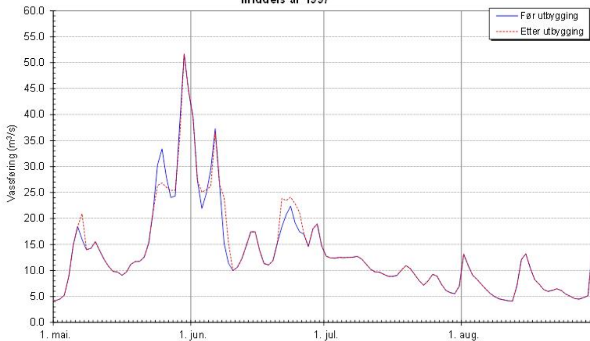
Gjengedal kraftverk. med reg av Storevatnet - Vassføring nedanfor kraftverket - middels år 1997
