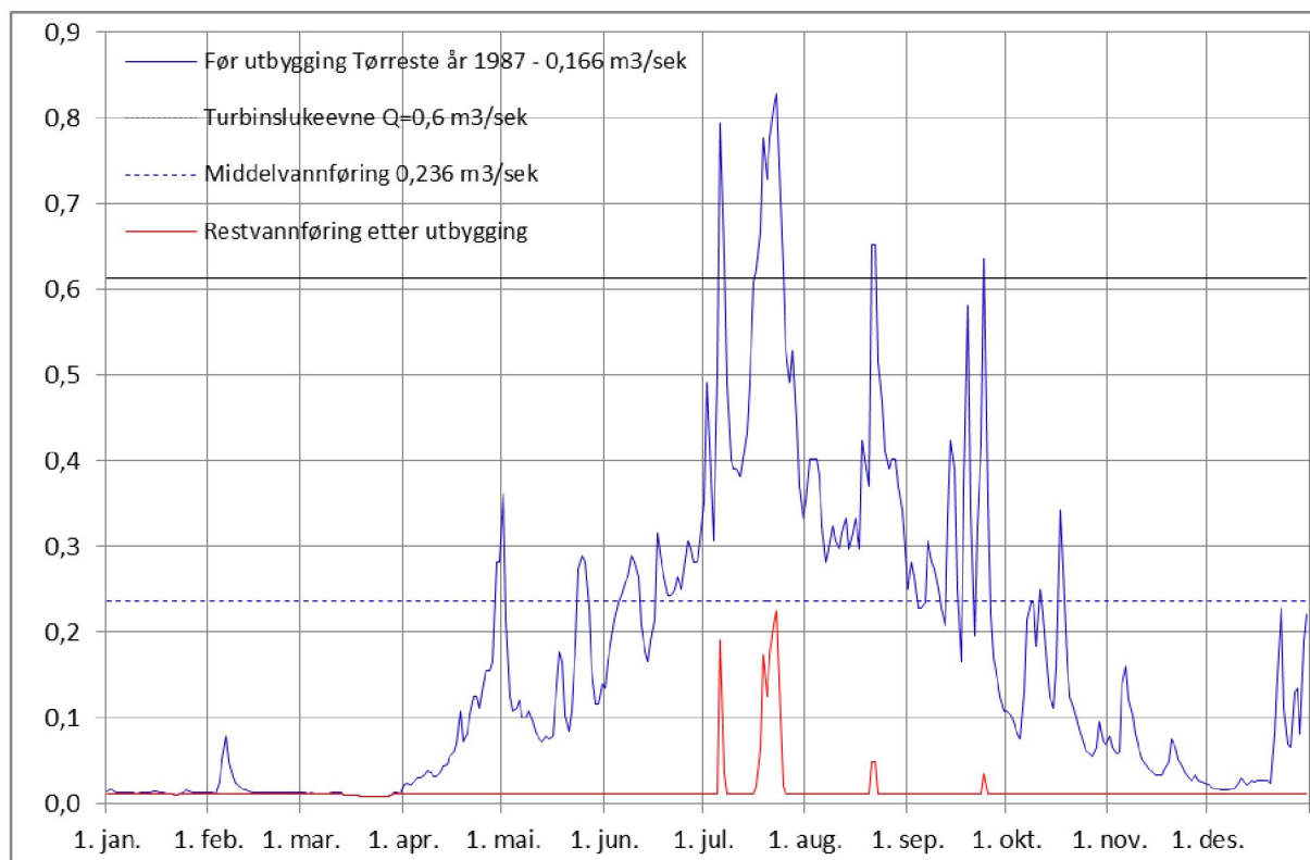
Figur 6 - Plott som viser vannføringsvariasjoner tørreste år (før og etter utbygging)
