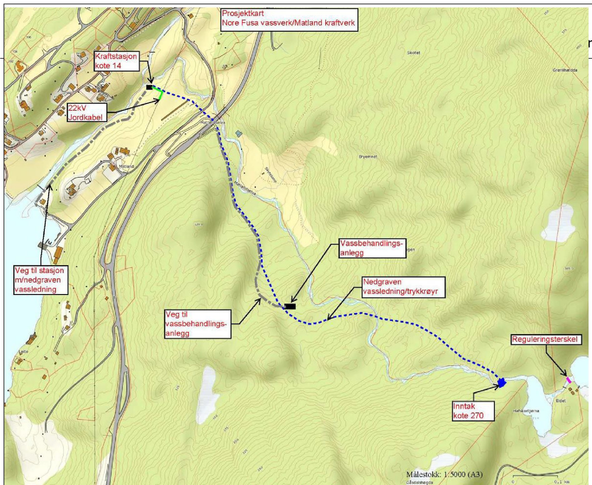
Fig. 9. Lokaliserte reguleringstiltak i Hafskorvatnet og Matlandselva, med dempingsmagasin, inntak, rørgate/vannledning, veier og kraftstasjon (14 moh). I tillegg vannbehandlingsanlegg for kommunalt vannverk. Kilde: Tiltakshaver.
