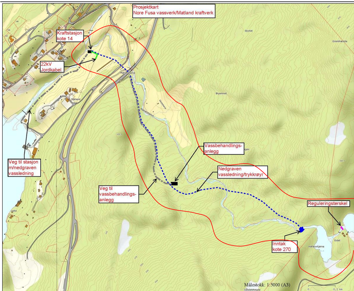
Fig. 9. Lokaliserte tiltak i Matlandselva, med inntak, rørgate, veier og kraftstasjon (14 moh). I tillegg anlegg for kommunalt vannverk. Et generelt influensområde på 100 meter ut fra påvirkede økosystem (akvatiske og terrestre) er vist. For Hafskorvatn, jfr. Fig. 10. Kartkilde: Tiltakshaver.
