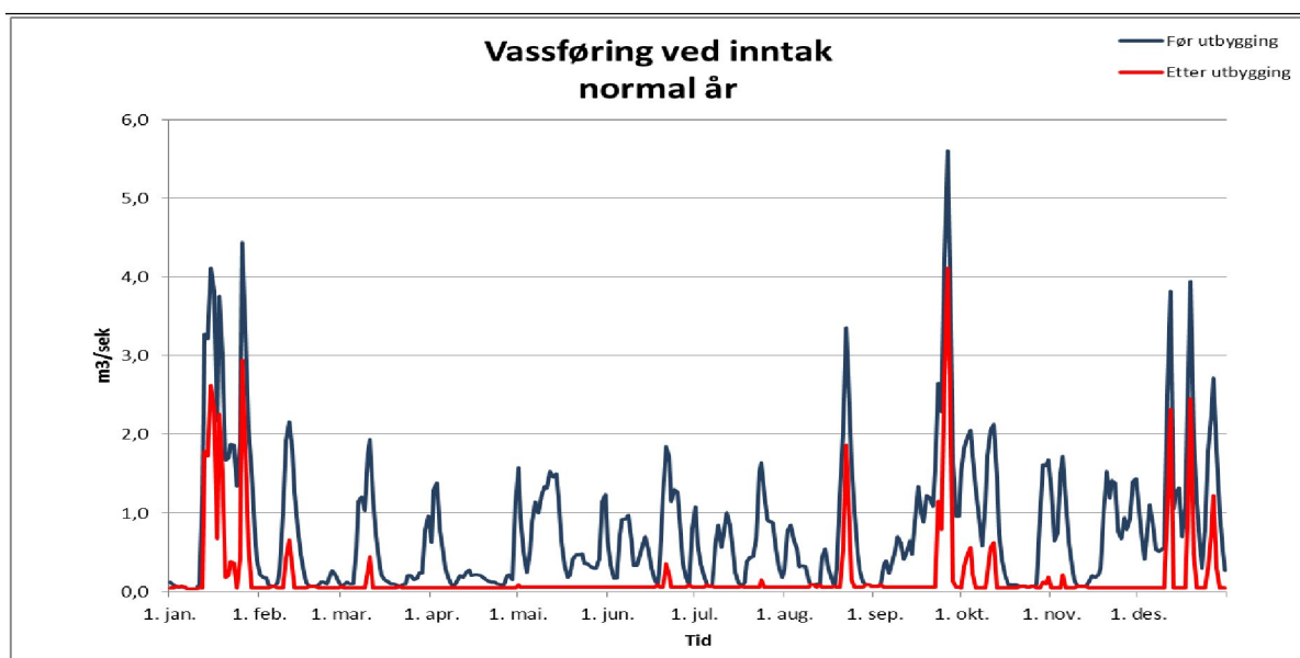
Fig. 53. Vannføring ( \text{m}^3/\text{s} ) i Matlandselva før og etter regulering i et normalår (2003). Kilde: SKL.
