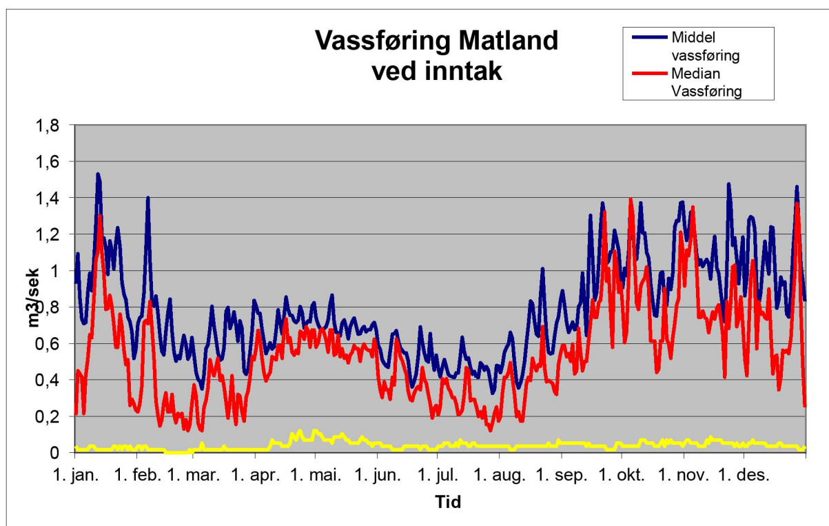
Fig. 7. Variasjon i vannføring i Matlandselva gjennom året, vist med middel vannføring, median vannføring og lavvannsføring.
