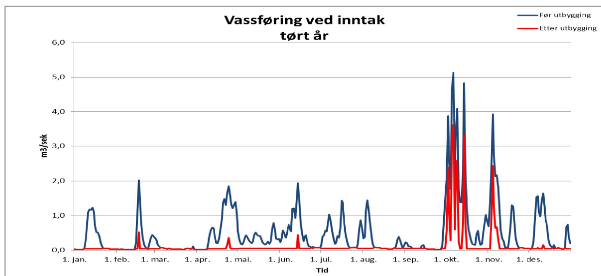
Fig. 54. Vannføring ( \text{m}^3/\text{s} ) i Matlandselva før og etter regulering i et tørt år (1996). Kilde: SKL.
