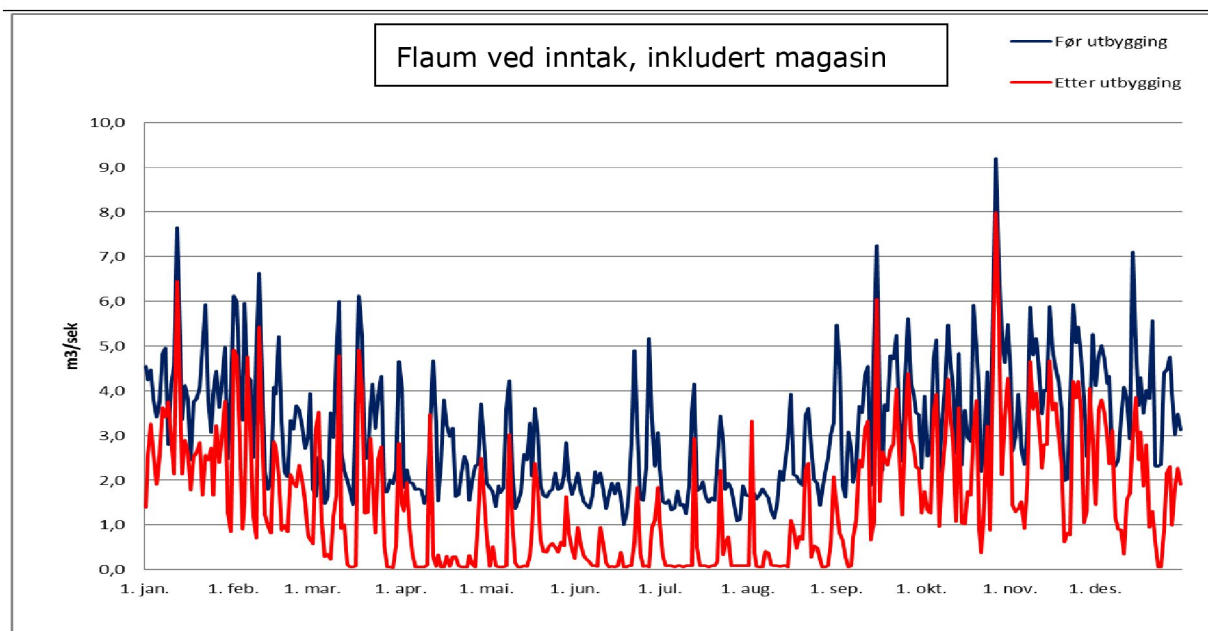
Fig. 56. Flomvannføring nedstrøms inntaket i Matlandselva før og etter regulering, med bruk av Hafskorvatnet som dempingsmagasin. Kilde: SKL.
