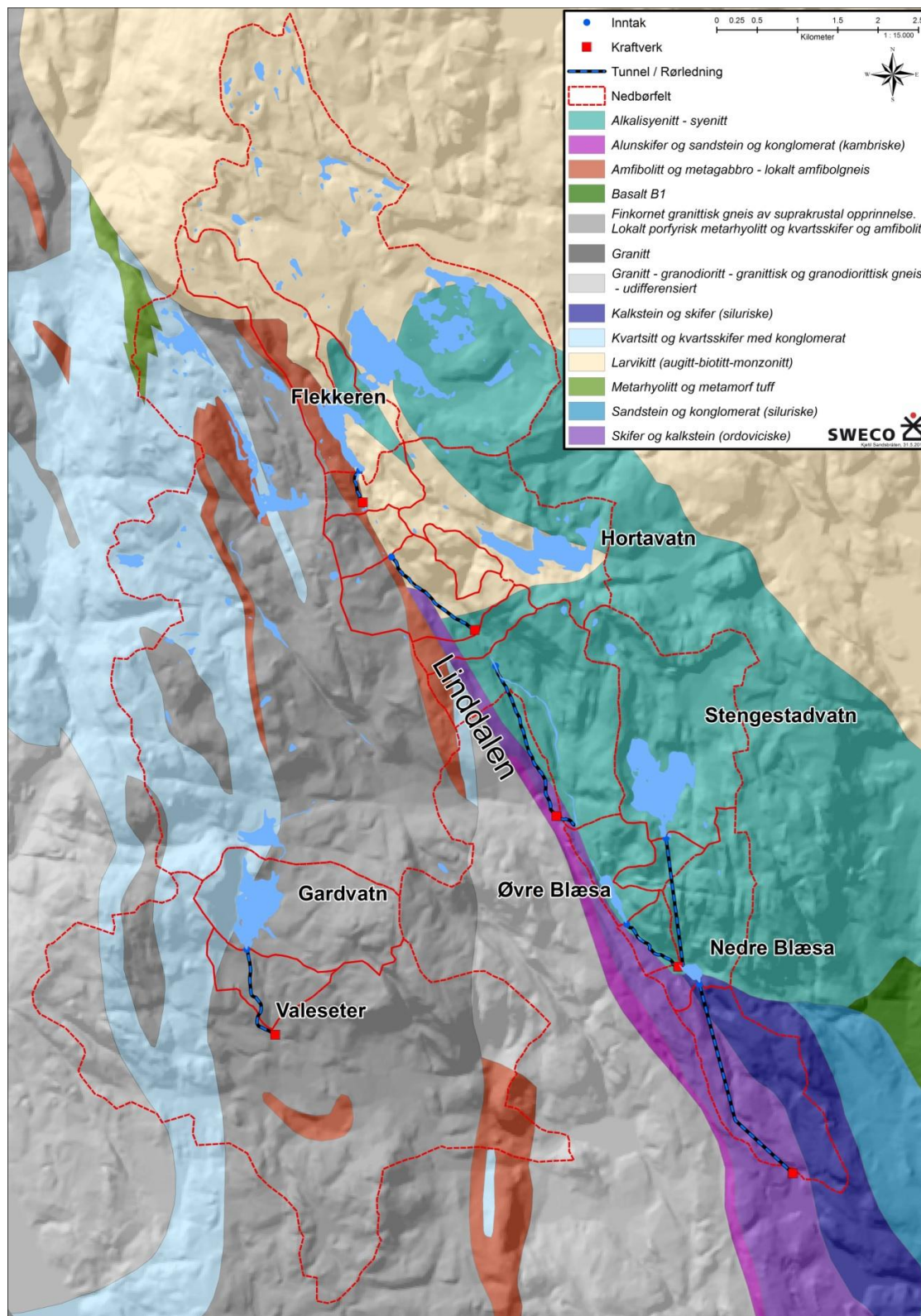
Figur 5-1Berggrunnsgeologien i området med inntegnet lokale nedslagsfelt for Linddalen og Gardvasselva (Kilde NGU). De nye kraftstasjonsprosjektene er inntegnet. For mer kartinformasjon se Figur 5-4 side18.
