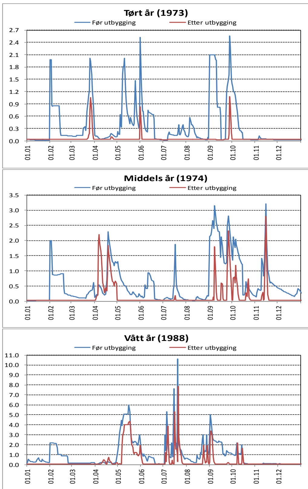
Figur 7-20 Vannføringer rett nedstrøms inntak Krosseter kraftverk i tre typiske år
