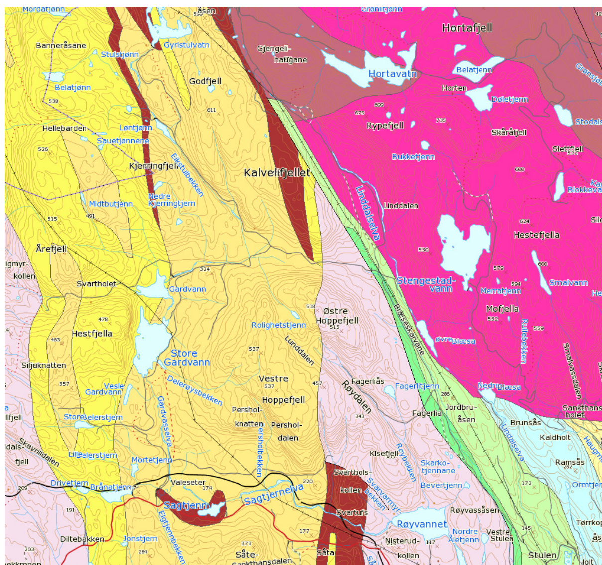
Figur 2. Berggrunnen i områdene fra Flekkerø vann i nord til Holt (Stulen) i sør og Gardvasselv og Valsester i vest (fra www.ngu.no/kart/arealisNGU ). Mørkt brunt: amfibolitt og metagabbro. Lyst brunt: larvikitt. Lyst grønt: skifer og kalkstein (ordoviciske). Lyst blått: kalkstein og skifer (siluriske). Rosa: alkalisyenitt – syenitt. Gul: finkornet granittisk gneis, lokalt med bl.a. kvartsskifer og amfibolitt. Grønt: Områder med bl.a. alunskifer og sandstein, men de er ikke innefor prosjektområdet.
