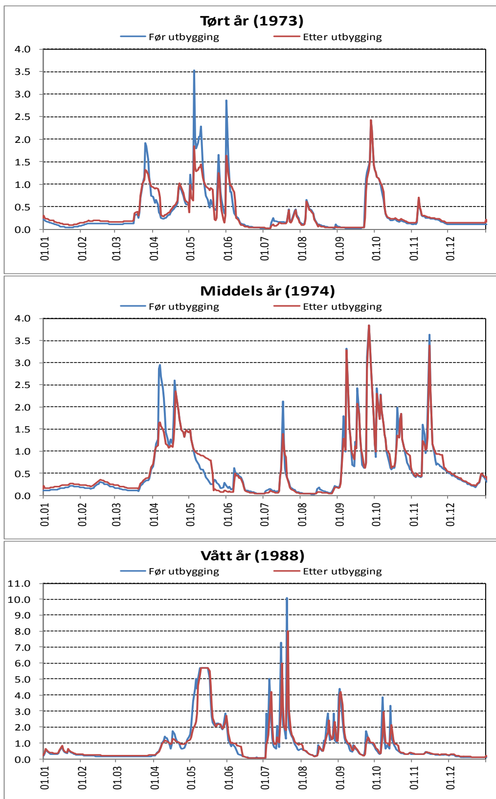
Figur 7-49 Vannføring i Bøelva ved utløpet i Røyvatn i tre typiske år
