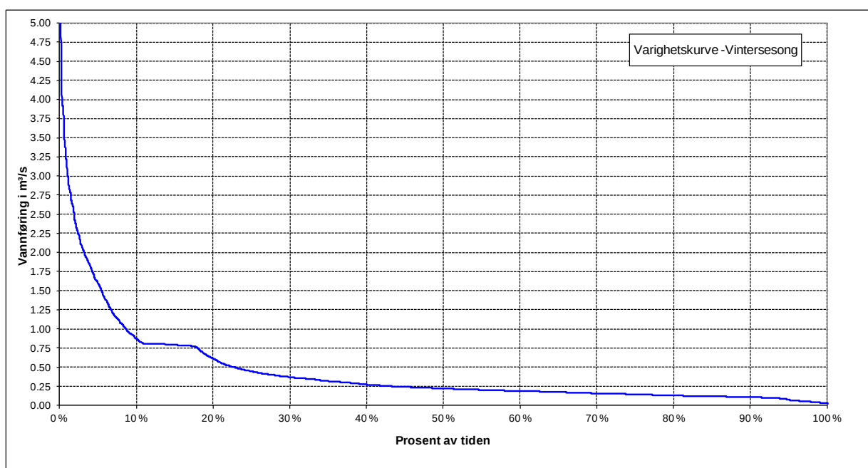
Figur 7-10 Varighetskurve vinter (1.10-30.4) for tilsig til Losmentmyra kraftverk
