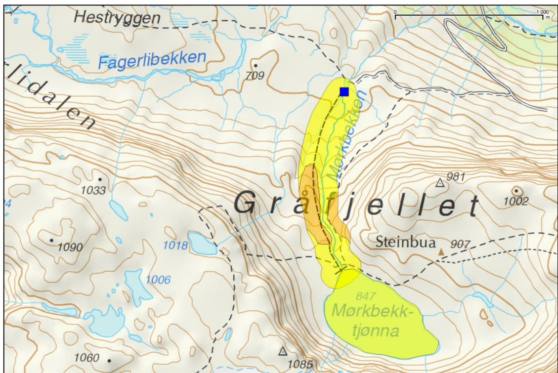
Figur 12. Verdikart over influensområdet. Områder med liten verdi med gul farge, mens områder med middels verdi har oransje farge. Det østlige området med middels verdi er estimert ut fra observasjoner av topografi og sedimentologi samt forekomst av basekrevende karplanter.
