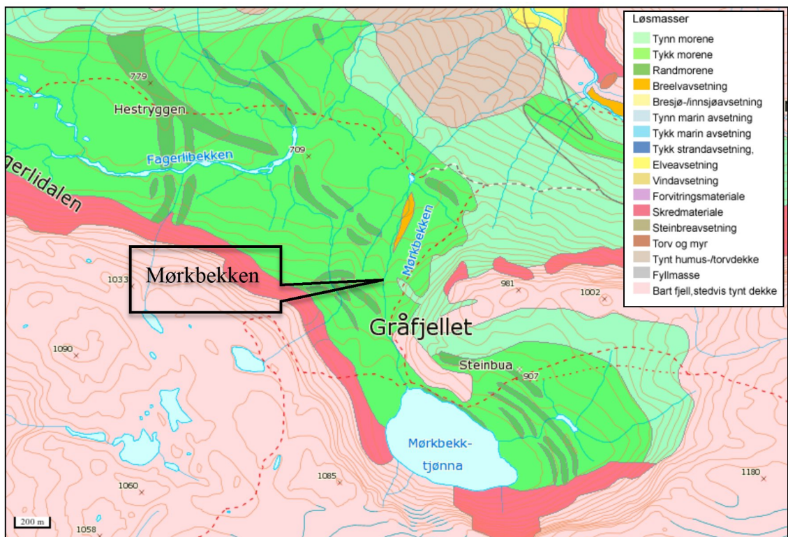
Figur 7. NGU's løsmassekart viser at influensområdet har mye tykk morene (grønn). Noe breeelvavsetninger finnes langs elva, samt randmorenebelter. Kilde: Norges geologiske undersøkelse.
