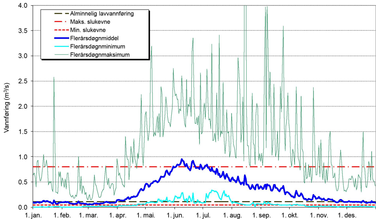
Figur 2-3 Daglige maksimumsvannføringer nedenfor inntak Høgseterelva for perioden 1973 - 2011.
