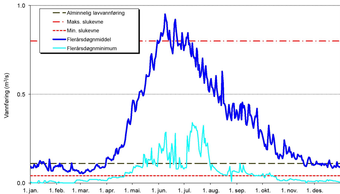
Figur 2-1 Minimum og middel på døgnbasis nedenfor inntak Høgsæterelva for perioden 1973 - 2011
