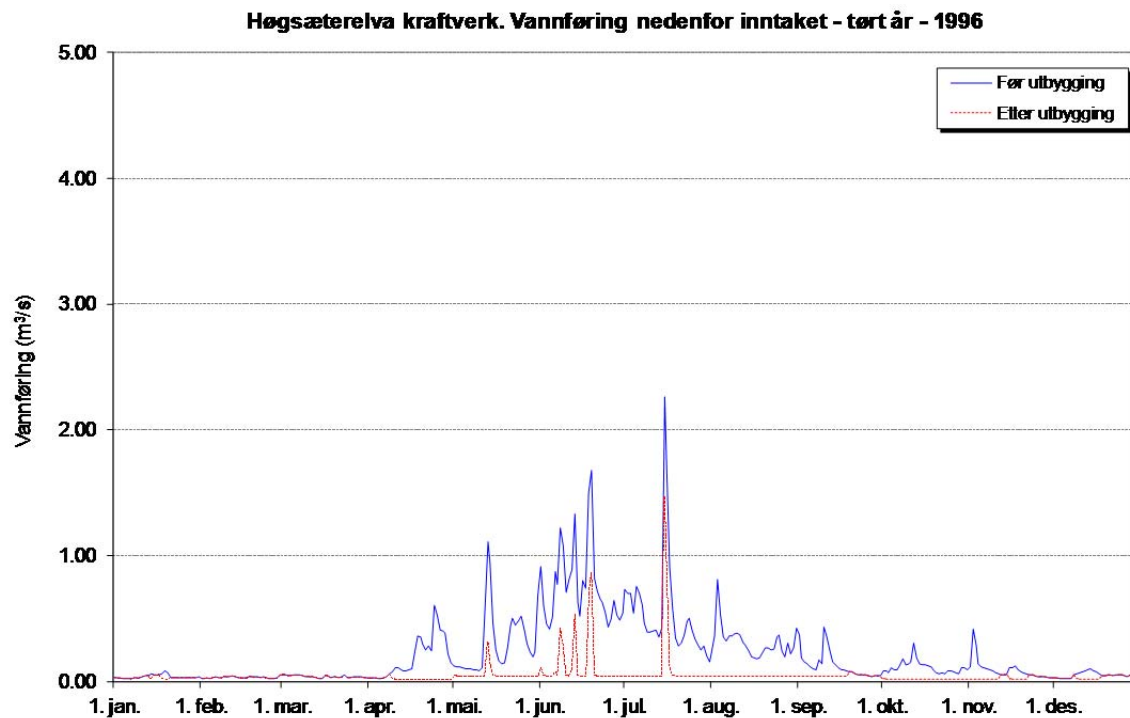
Figur 3: Vannføring like nedstrøms inntaket før og etter utbygging tørt år.
