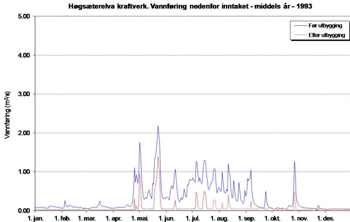
Figur 2: Vannføring like nedstrøms inntaket før og etter utbygging middels år.
