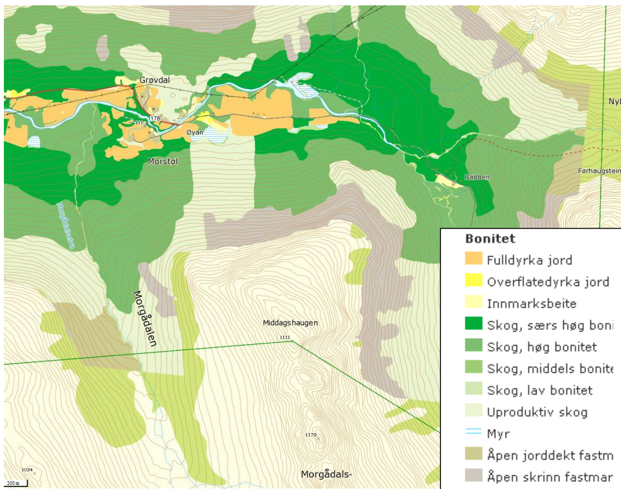
Figur 3-9 bonitetskart
