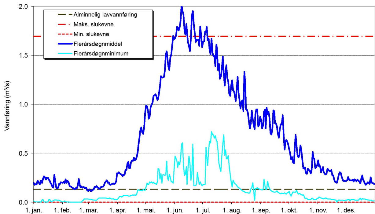
Figur 2-2 Minimum og middel på døgnbasis nedenfor inntak Rabbelva for perioden 1973 - 2011
