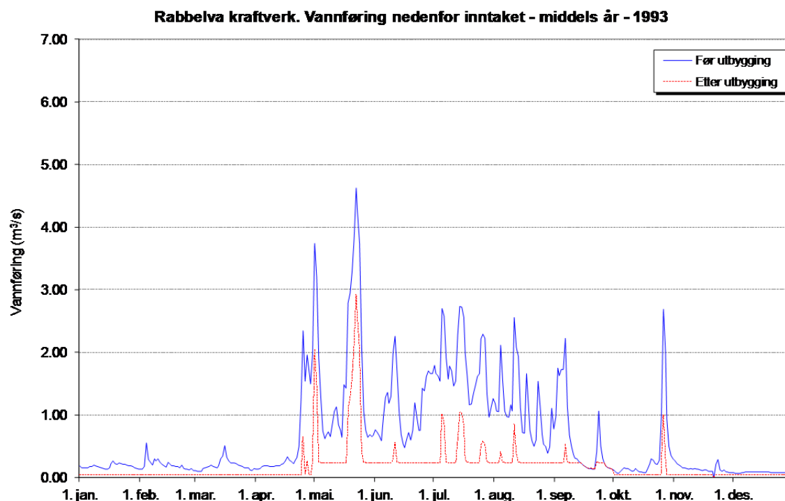
Figur 5: Vannføring Rabbelva like nedstrøms inntaket før og etter utbygging middels år.
