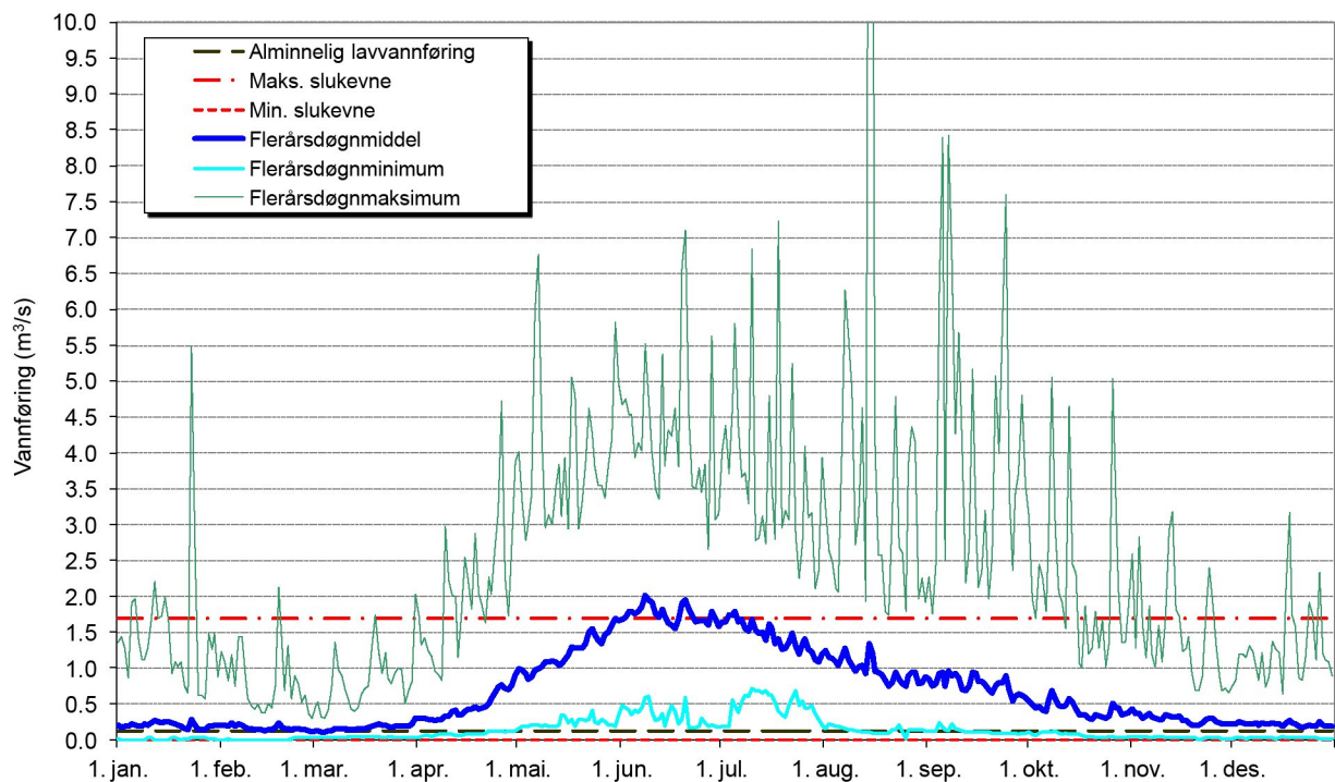
Figur 2-4 Daglige maksimumsvannføringer nedenfor inntak Rabbelva for perioden 1973 - 2011.
