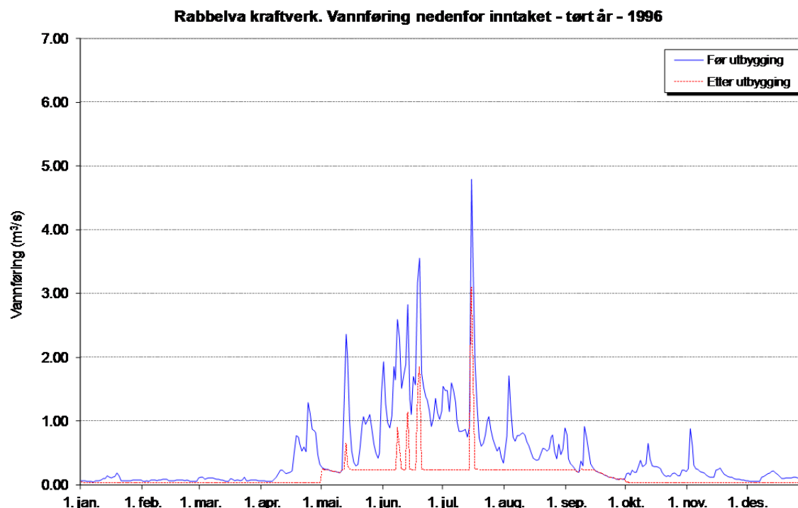
Figur 4: Vannføring Rabbelva like nedstrøms inntaket før og etter utbygging tørt år.
