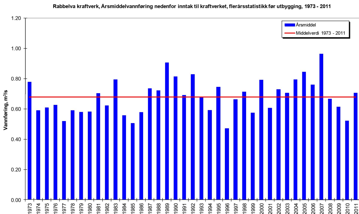
Figur 2-6 Middelvannføring hvert år for perioden 1973 - 2011 nedenfor inntak Rabbelva.
