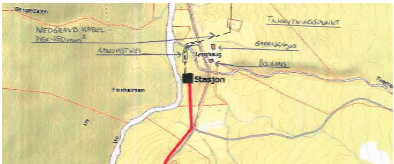
Nettilknytning Øvre Tømmerelv kraftverk vist med stiptet linje
