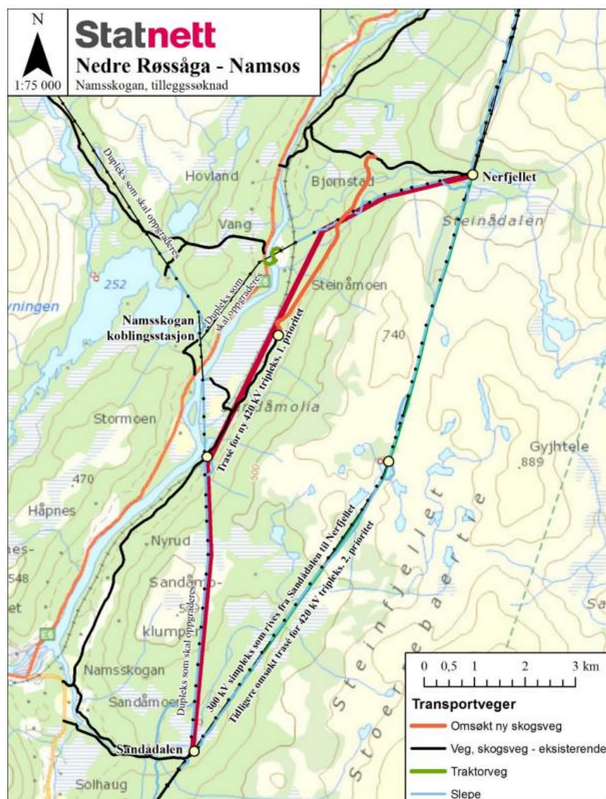
Figur 3-3 Kart hentet fra Statnetts konsesjonssøknad. Den østre ledningstraséen mellom Nerfjellet og Sanddalen (blå farge) er dagens trasé, og den opprinnelig omsøkte traséen. Dette er endret slik at den vestre om Namsskogan koblingsstasjon blir valgt (rød farge på kartet).
