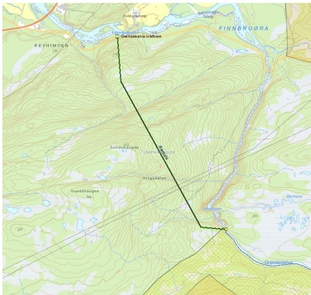
Figur 4-5 Grøndalselva kraftverk. Adkomstvei til kraftverket bygges i forlengelse av skogsbilvei neders til høyre på kartet. FV764 i overkant av kartet og E6 går øverst til venstre. Drivlei og oppsamlingsområde for rein i nedkant av kartet.
