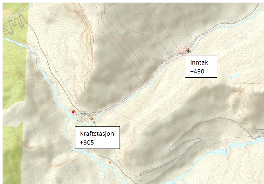
Fig. 13 Teknisk plan
