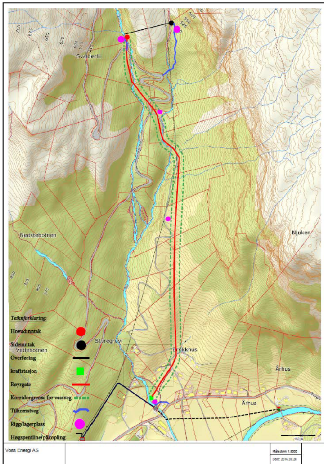
Fig. 4 Oversikt over planlagte installasjonar og arealbeslag i samband med bygging av Storagroe kraftverk. Den store elva til høgre i nedste del av kartet er Teigdalselvi.
