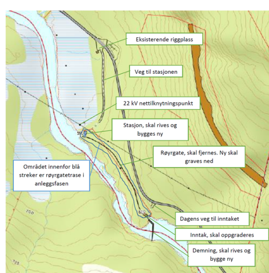
Fig. 29 Dagens anlegg (til høgre) skal rustast opp som vist på kartet til venstre. I verna vassdrag kan konsesjon for kraftverk opp til 1 MW og opprusting av eksisterande anlegg vurderast om tiltaket ikkje
