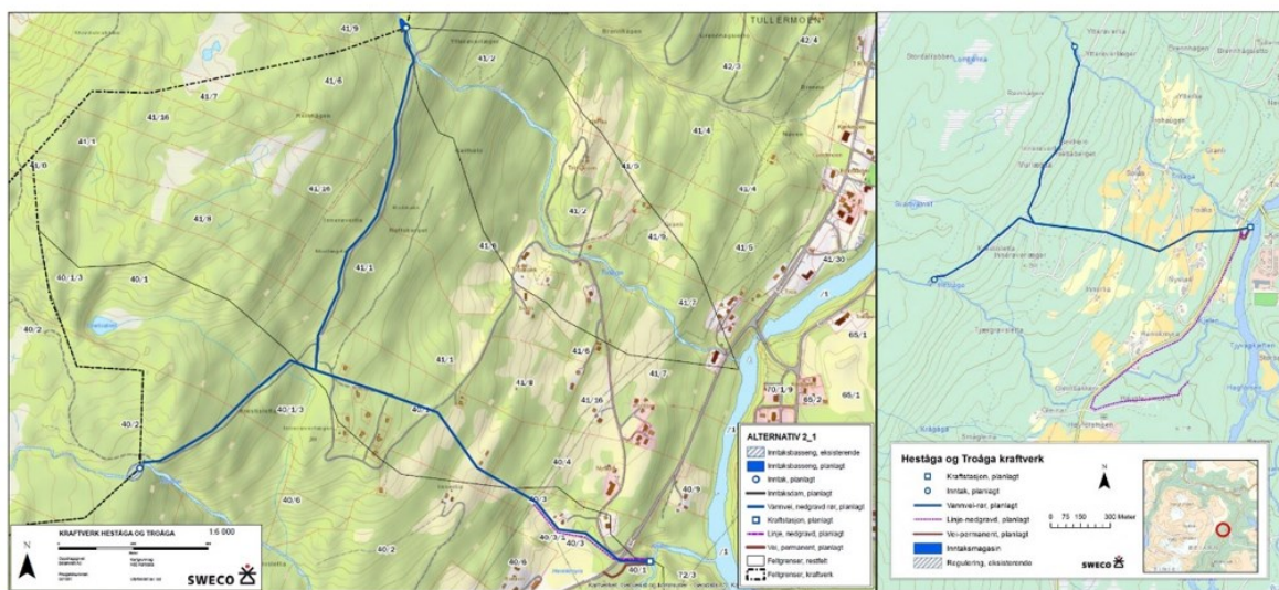
Figur 3 viser ny prosjektskisse av Heståga/Troåga kraftverk til venstre, og opprinnelig prosjektskisse til høyre.
